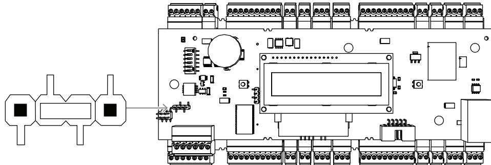
Figura 4.12: Configuración para la conexión RS-485 con cuatro cables
