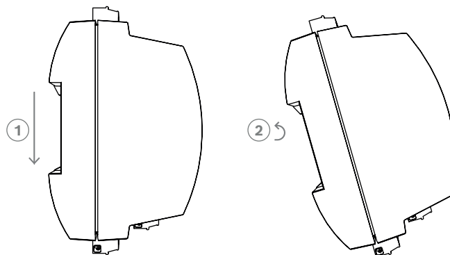
Figura 4.2: Desmontaje del controlador del carril de montaje
