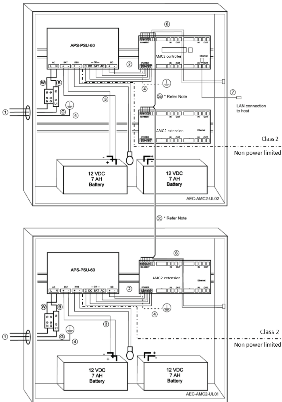
Figura 6.1: Ejemplo de montajes con ampliaciones
