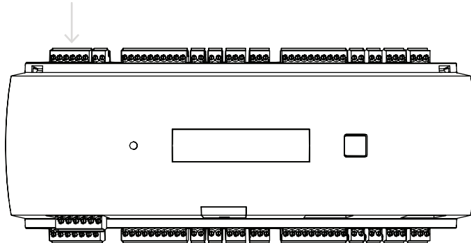
Figura 4.14: Ubicación del bus del módulo de ampliación RS-485
