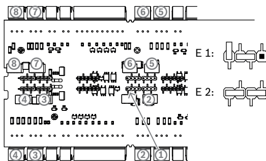
Figura 4.20: Ubicación de los puentes de la salida de relé (parte inferior)
