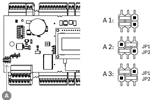
Figura 4.5: Ubicación de la interfaz de host de RS-485 del puente con toma de tierra
