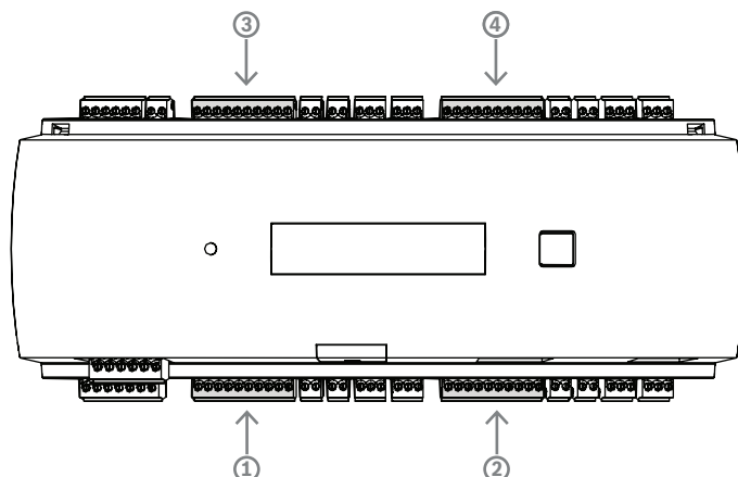
Figura 4.16: Ubicación de la interfaz Wiegand (puerto) para lectores
