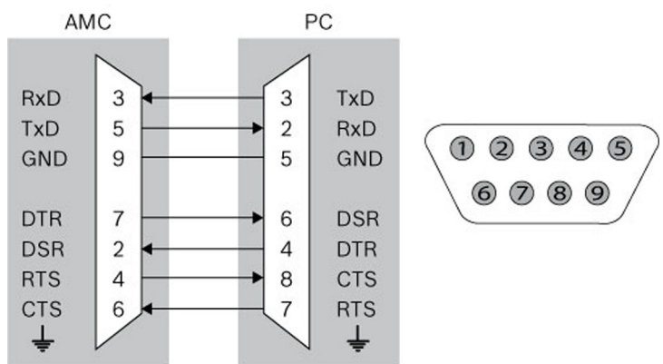
Figura 11.2: Diagrama de interconexión de la interfaz específica del proyecto
