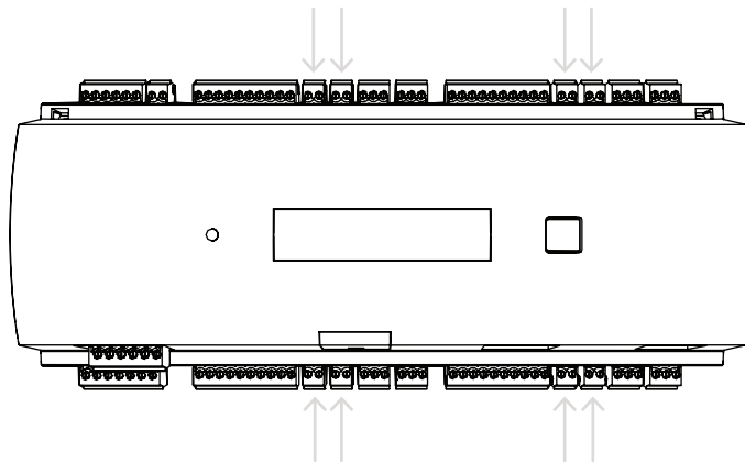
Figura 4.21: Ubicación de los conectores de entrada analógica
