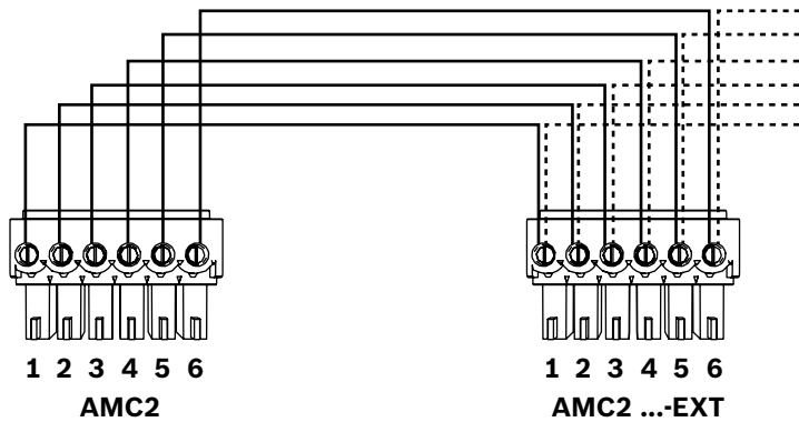
Figura 4.15: Conexión de un módulo de ampliación a un AMC2
