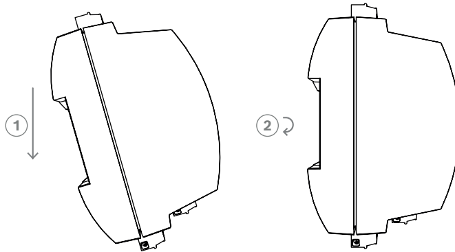
Figura 4.1: Montaje del controlador en un carril de montaje
