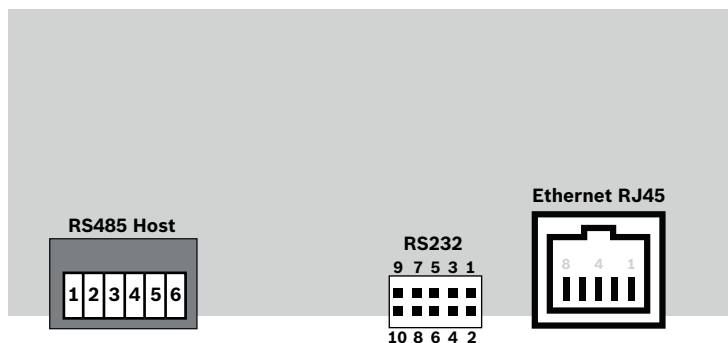
Figura 11.1: Conectores en PCB superiores La interfaz RS-485 no es compatible con: - BIS 4.9.1 y posteriores - AMS 4.0 y posteriores.
