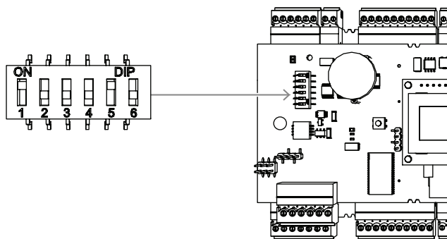
Figura 7.2: Interruptores DIP y estado de entrega
