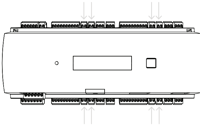
Figure 4.21: Emplacement des connecteurs d'entrée analogique
