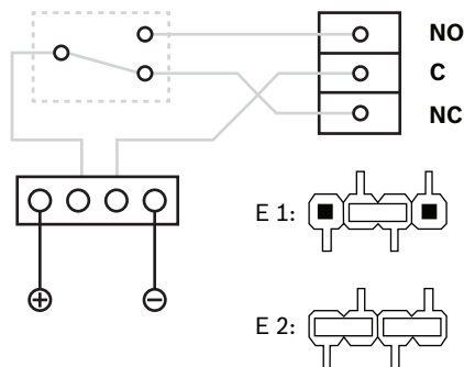
Figure 4.18: Paramètres du mode relais
