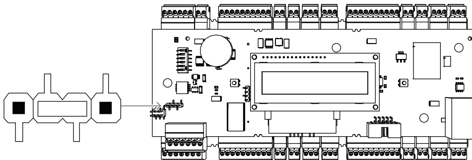
Figure 4.12: Paramètres pour une connexion RS-485 à quatre fils Sélectionnez l'adresse RS-485 du contrôleur AMC2 à l'aide du commutateur DIP.
