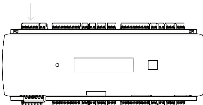
Figure 4.14: Emplacement du bus du module d'extension RS-485
