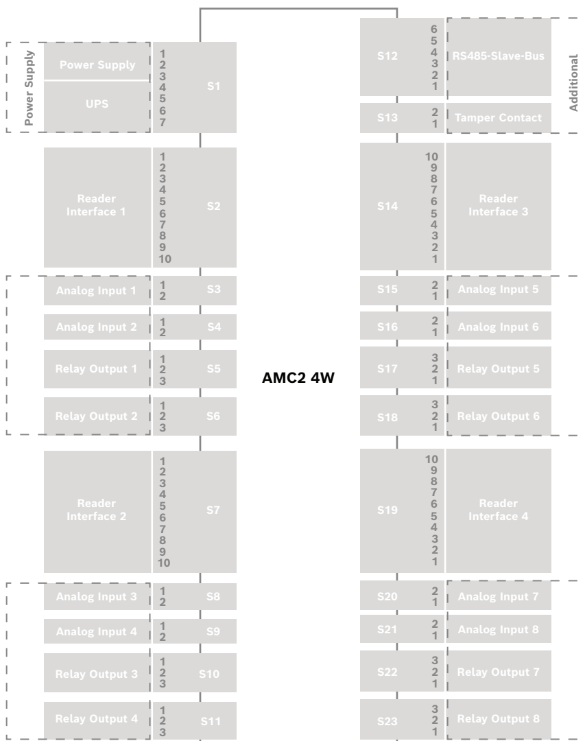
Figure 11.3: Borniers de l'AMC2-4W
