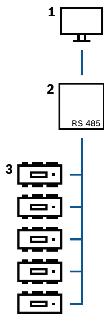
Figure 4.9: Configuration d'un système hôte RS-485
