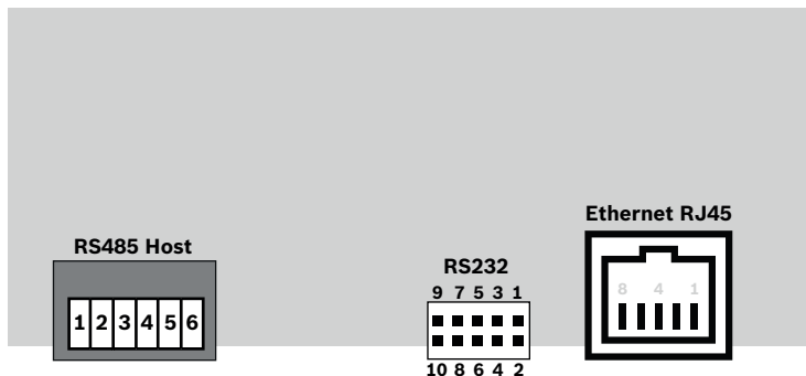
Figure 11.1: Connecteurs sur la carte PCB supérieure L'interface RS-485 n'est pas prise en charge par :
