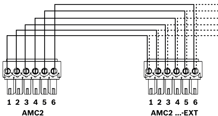
Figure 4.15: Connexion d'un module d'extension à un contrôleur
