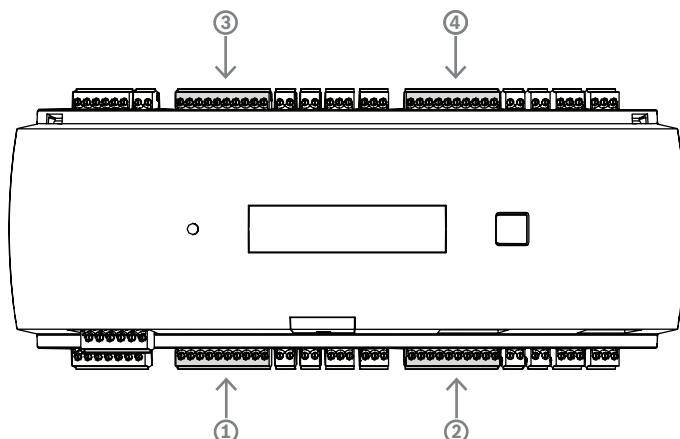
Figure 4.16: Emplacement de l'interface Wiegand (port) pour les lecteurs
