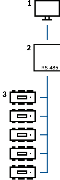
Şekil 4.9: RS-485 ana bilgisayar sisteminin yapılandırması
