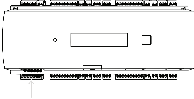
Şekil 4.7: Güç kaynağı konnektörünün konumu
