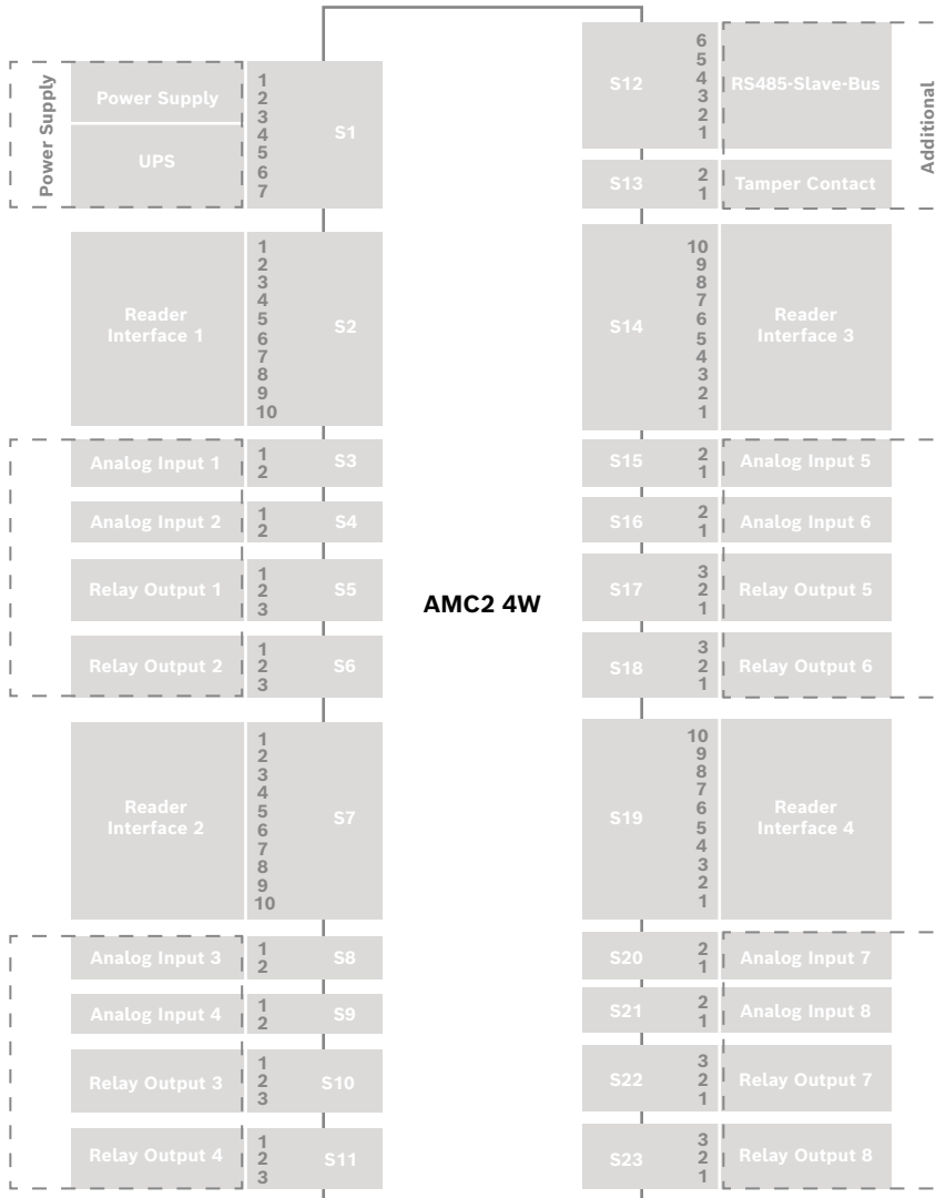
Şekil 11.3: AMC2-4W konnektör blokları
