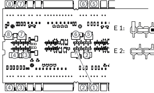
Şekil 4.20: Röle çıkış atlama tellerinin konumu (alt taraf)
