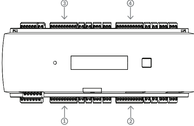
Şekil 4.16: Okuyuculara ait Wiegand arayüzünün (port) konumu
