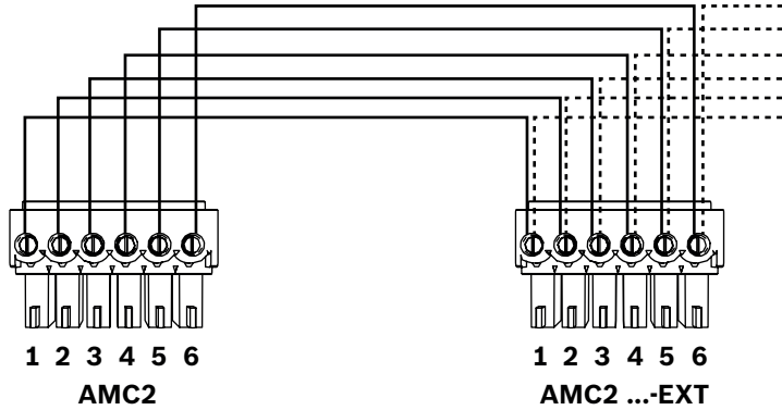
Şekil 4.15: Geniřletme modülünün AMC2 bağlantısı
