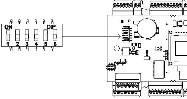
Şekil 4.13: Ana bilgisayar ayarları ve teslimat durumu için seçicinin konumu
