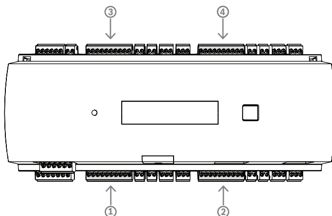
图片 4.16: 读卡器Wiegand接口（端口）的位置
