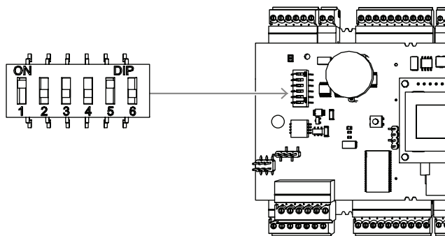
图片 4.13: 主机设置和传输状态选择器的位置
