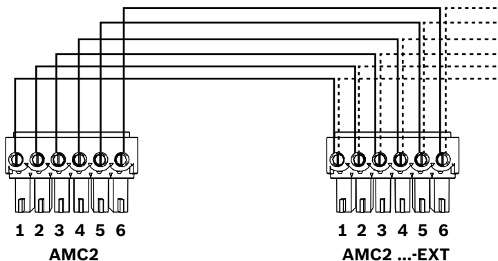
图片 4.15: 将扩展模块连接到控制器
