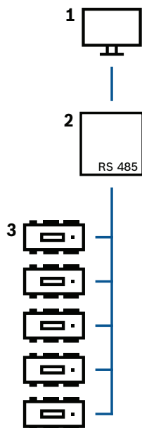
图片 4.9: RS-485主机系统的配置
