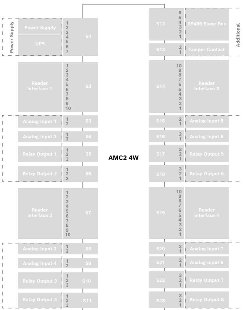
图片 11.3: AMC2-4W 的连接器座
