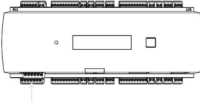
图片 4.7: 电源设备连接器的位置
