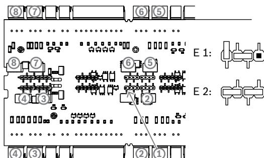
图片 4.20: 继电器输出跳线（底部）的位置
