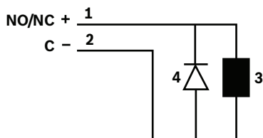
图片 4.19: 恢复二极管示意图
