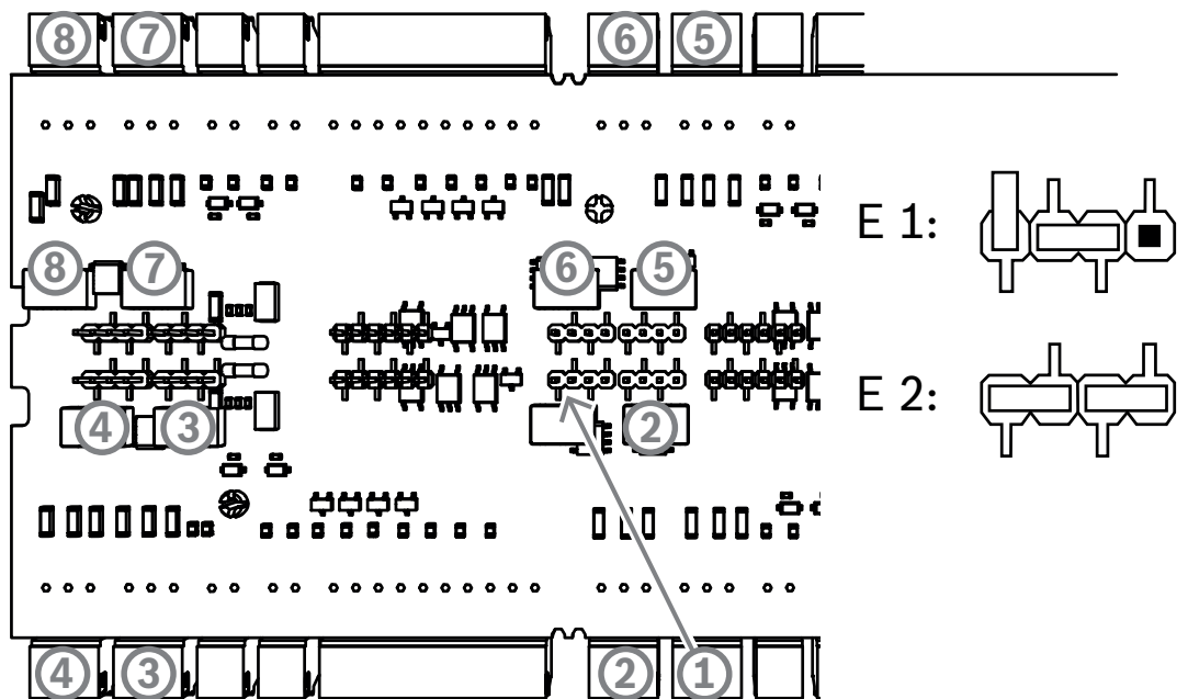
Abbildung 4.10: Position der Jumper für die Relaisausgänge
