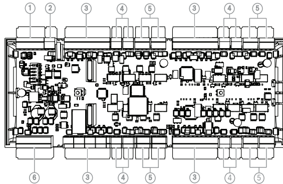
Abbildung 3.2: Übersicht – Schnittstellen
