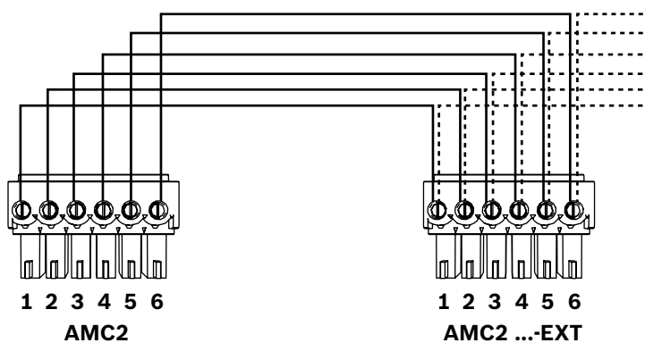
Abbildung 4.6: Anschluss eines Erweiterungsmoduls an einen Controller
