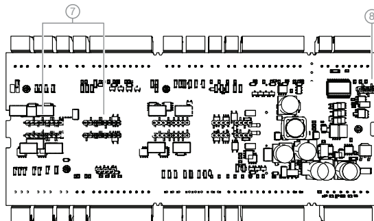
Abbildung 3.3: Jumper auf der Unterseite
