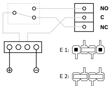
Abbildung 4.8: Einstellungen für den Relaismodus
