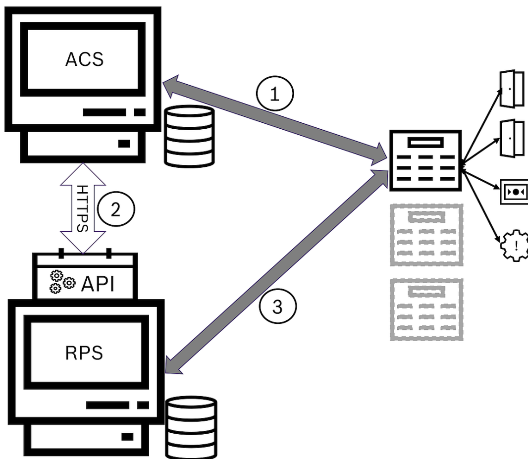
Figure 10.1: Topologie simplifiée du système ACS-Intrusion
