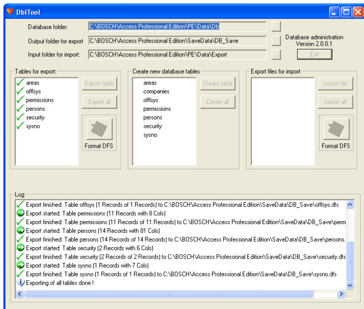
Figure 5.2: Désinstallation - Exportation de la base de données
