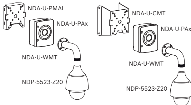
Fig. 3: Montage sur poteau (IP66) ; Montage en angle (IP66)
