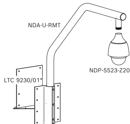
Fig. 4: Montage parapet (IP66) *En option pour montage parapet à plat
