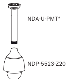
Fig. 2: Montage suspendu plafond *NDA-U-PMTE : tube d'extension 50 cm en option
