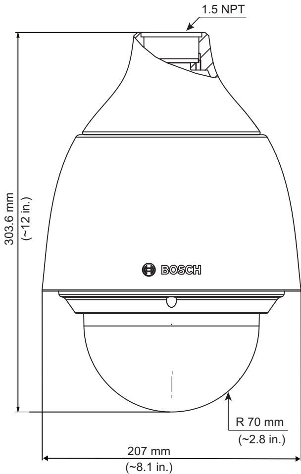
그림 7: 펜던트형 모델
