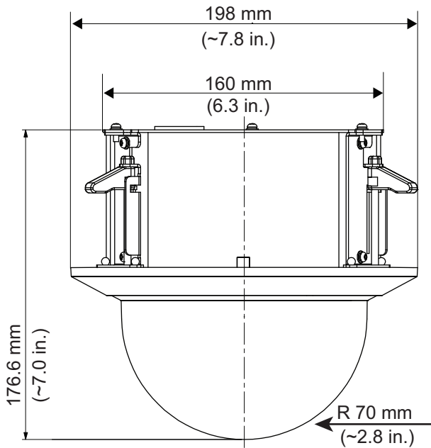
그림 6: 천장내 매립식 모델
