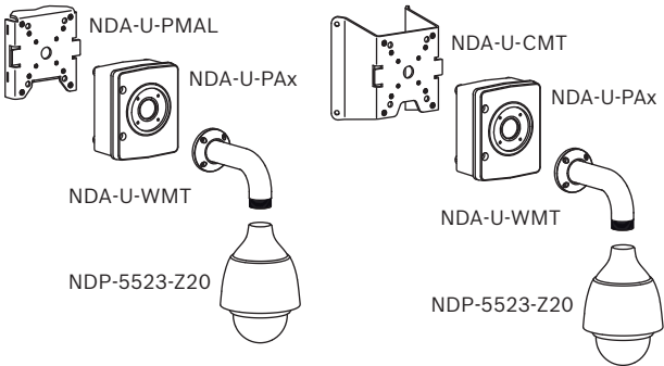
그림 3: 기둥 장착(IP66); 코너 장착 (IP66)
