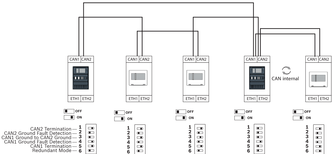
Figura 10.5: Ajustes de los conmutadores DIP para el lazo con teclado remoto (solo AVENAR)
