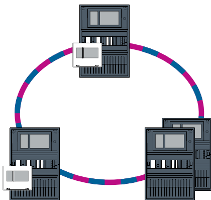
Figura 4.3: Lazo Ethernet
