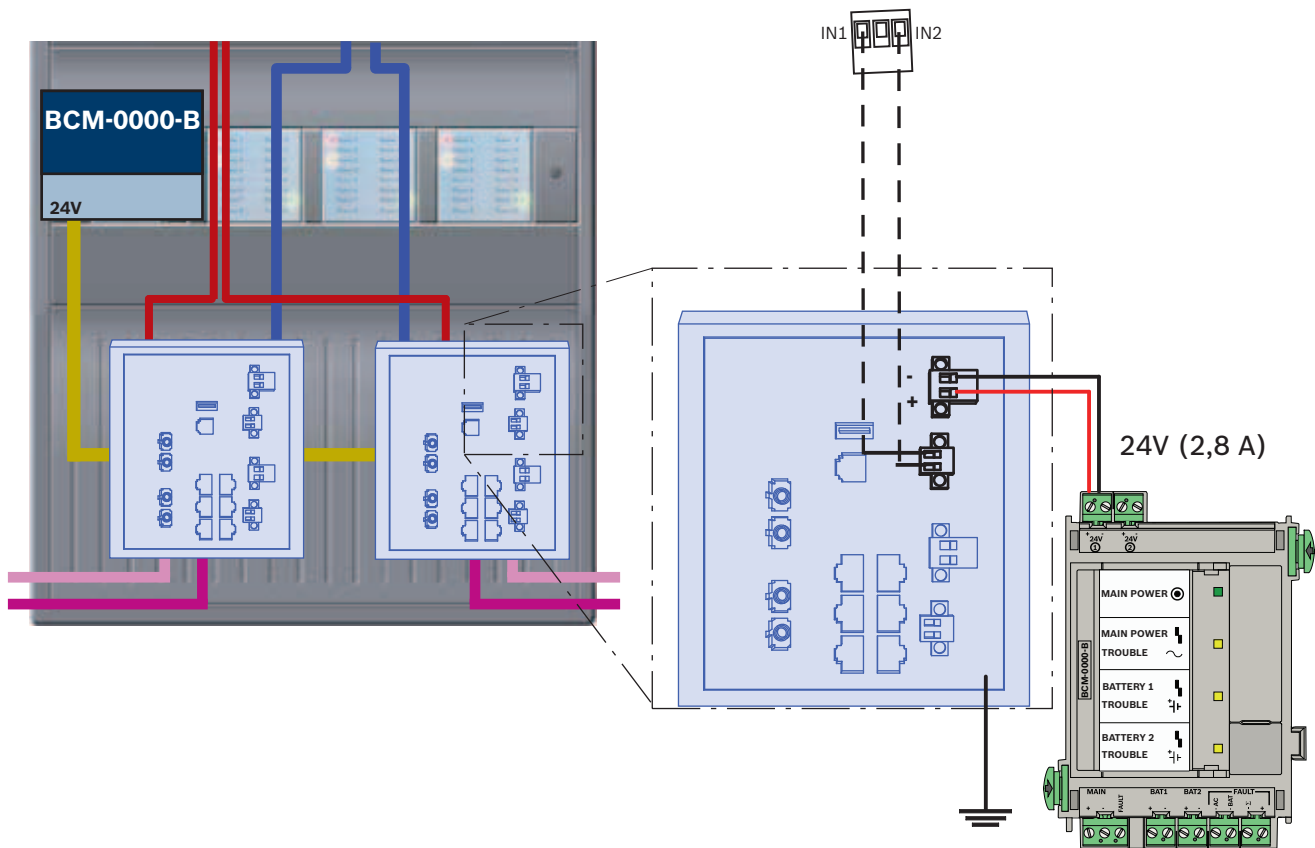
Figura 11.3: Conexión del conmutador a la fuente de alimentación y al controlador de la central
