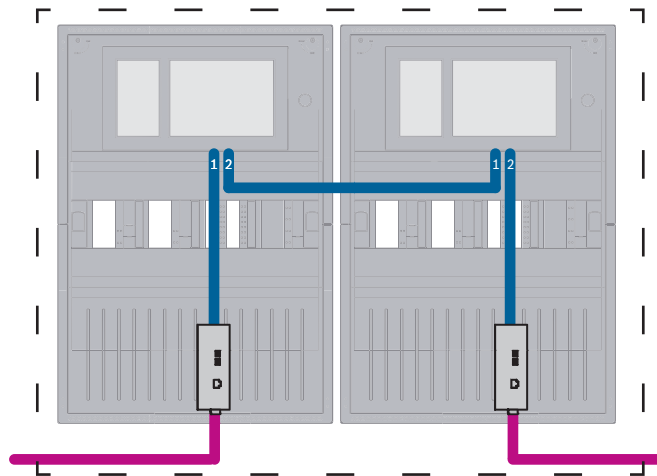
Figura 7.4: Red de centrales sobre Ethernet con centrales redundantes
