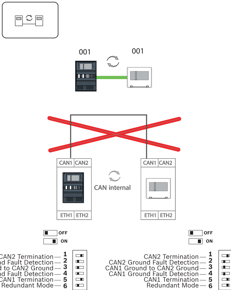
Figura 10.2: Ajustes de los conmutadores DIP para el teclado remoto como central redundante (solo AVENAR)
