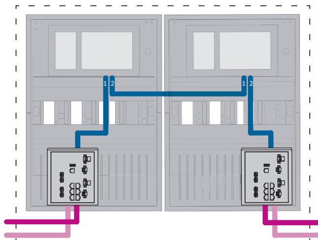
Figura 7.7: Conectar redes Ethernet con centrales redundantes
