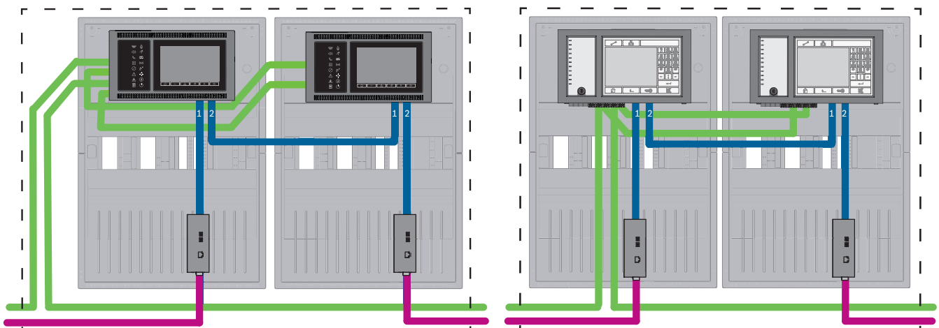
Figura 7.8: Conectar redes Ethernet y CAN con centrales redundantes
