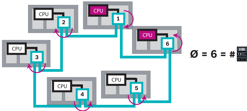
Figura 5.2: Diámetro de red de un lazo con 6 centrales
