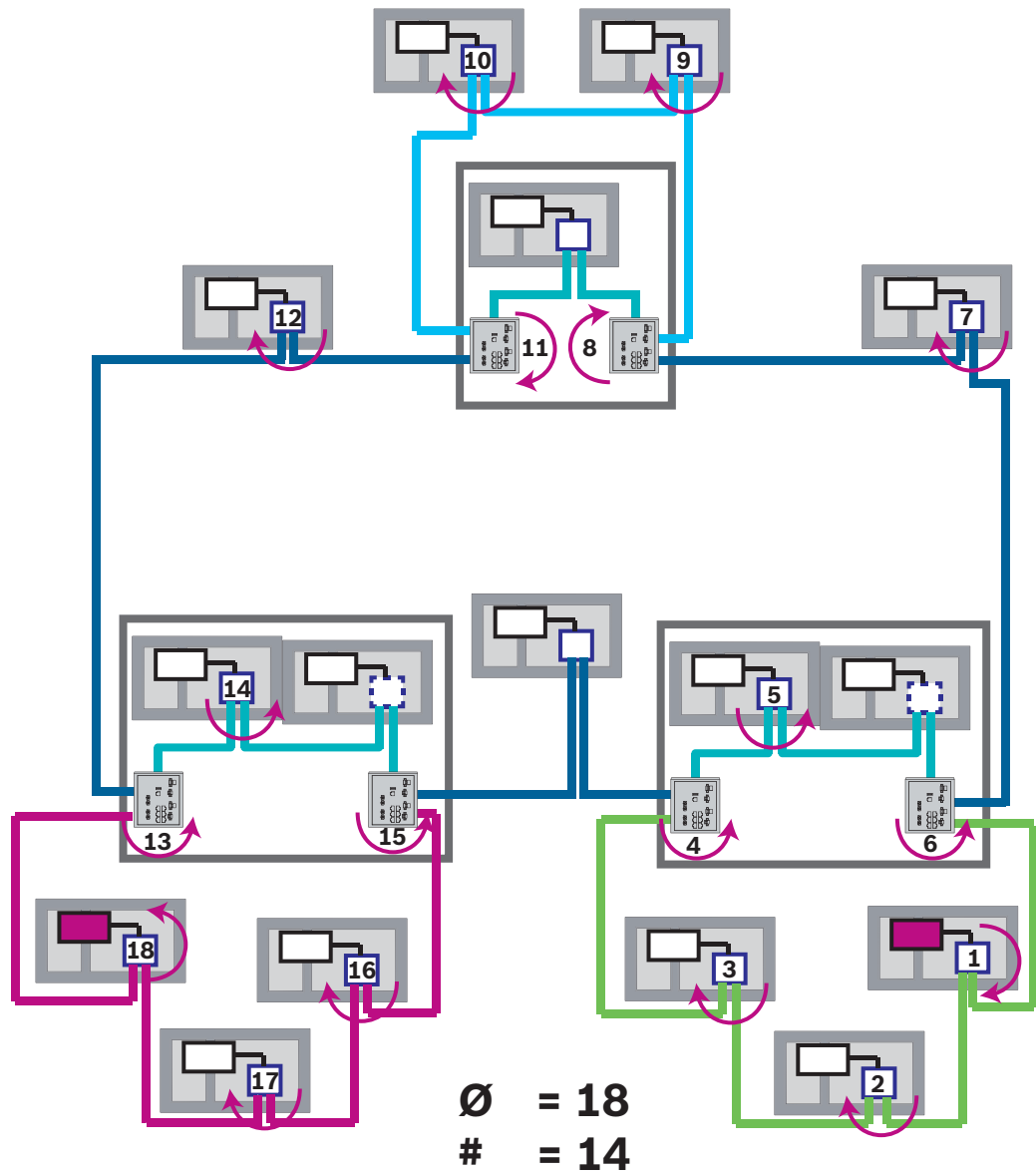
Figura 5.3: Diámetro de una red troncal con lazos secundarios La figura muestra el diámetro que tiene para encontrar la ruta más larga.
