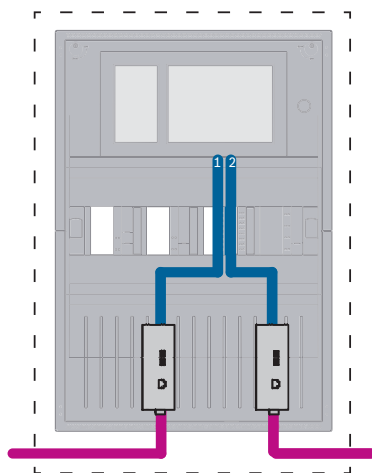
Figura 7.1: Red de centrales sobre Ethernet
