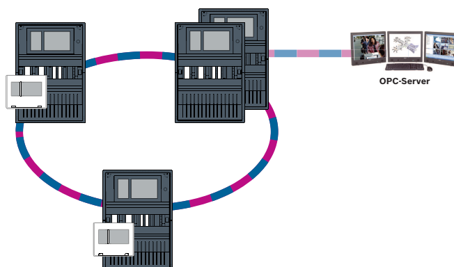
Figura 4.5: Lazo Ethernet con servidor OPC a una central redundante
