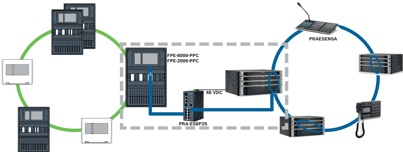
Figura 9.2: PRAESENSA a AVENAR panel
