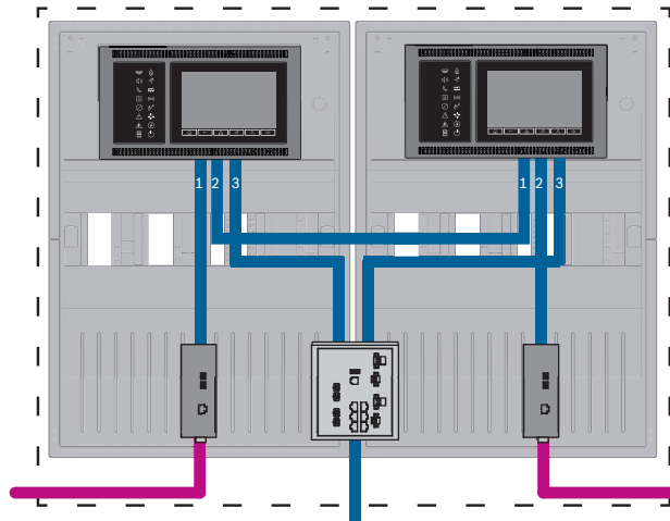
Figura 7.11: Módulo de central jerárquica y VAS a AVENAR panel redundante
