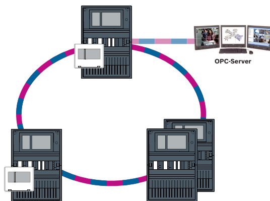
Figura 4.4: Lazo Ethernet con servidor OPC
