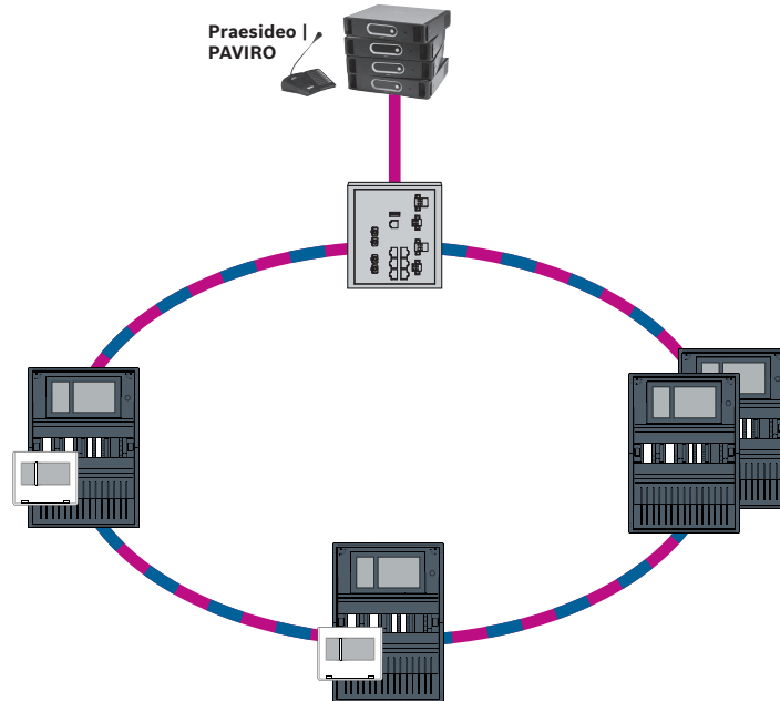
Figura 9.4: VAS integrada en red de central Ethernet
