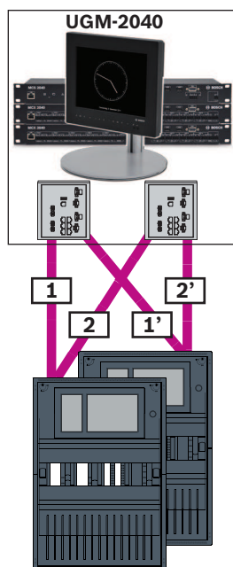
Figura 12.2: Ejemplo de numeración de líneas para el UGM-2040
