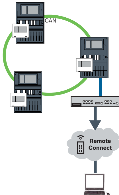
Figura 8.2: Remote Connect en un lazo CAN
