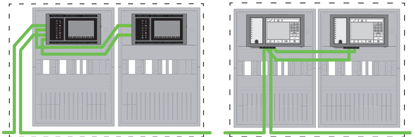
Figura 7.5: Red de centrales sobre CAN con centrales redundantes
