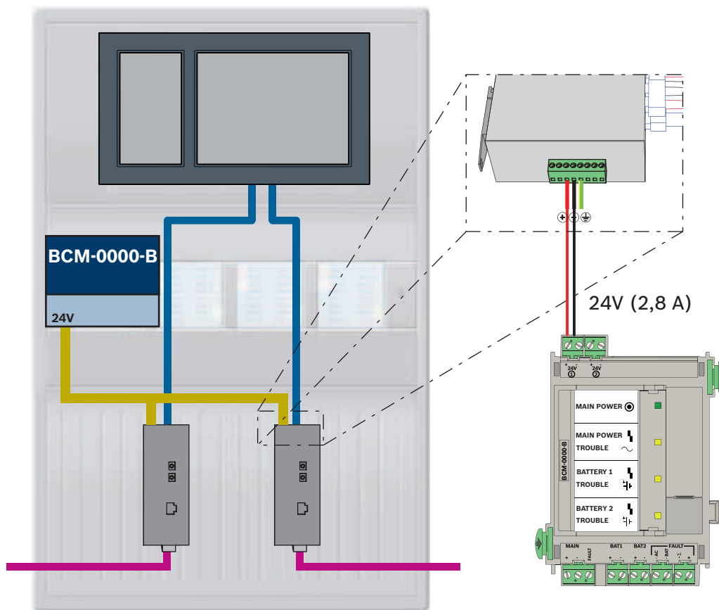
Figura 11.1: Conexión del convertor de medios a la fuente de alimentación y al controlador de la central IN1/IN2
