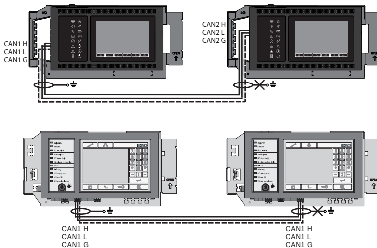
Figura 6.1: Conexión a CAN (superior: AVENAR, inferior: FPA)
