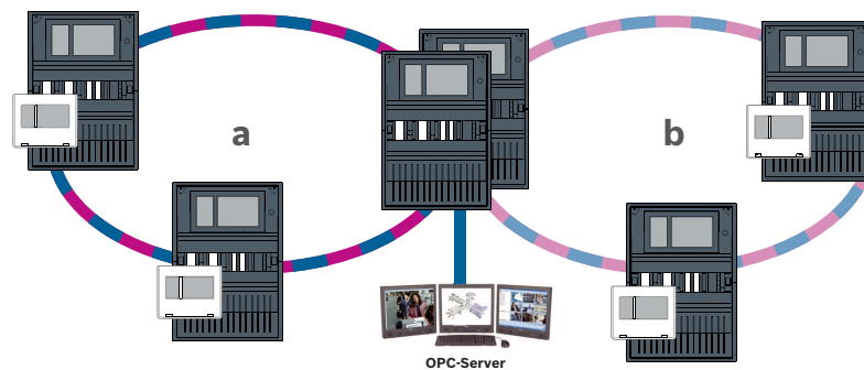
Figura 4.10: Conexión de un lazo Ethernet a través de una central redundante
