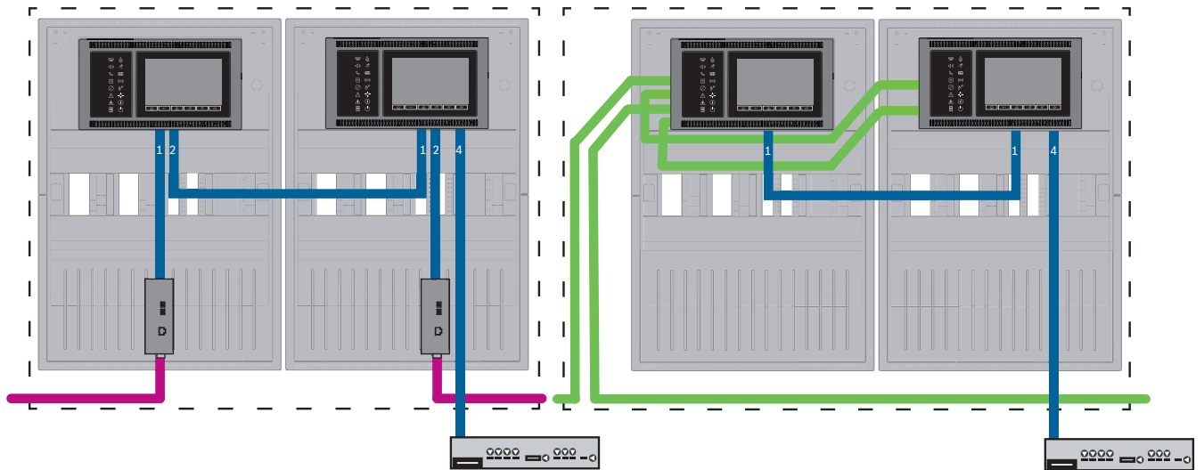
Figura 7.9: Lado izquierdo: en red Ethernet Lado derecho: en red CAN
