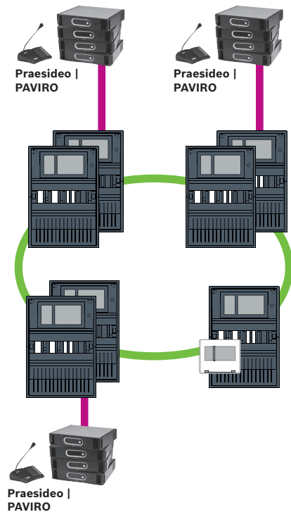
Figura 9.3: Varios módulos VAS directos
