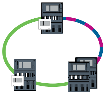
Figura 4.7: Bucle CAN con segmentos Ethernet
