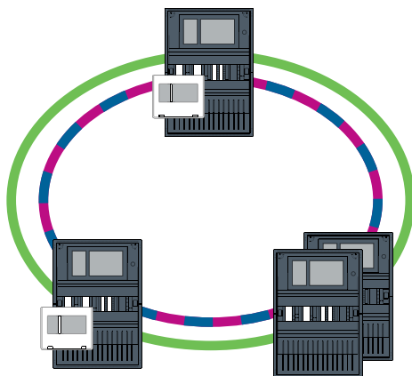
Figura 4.6: Lazo doble de Ethernet y CAN
