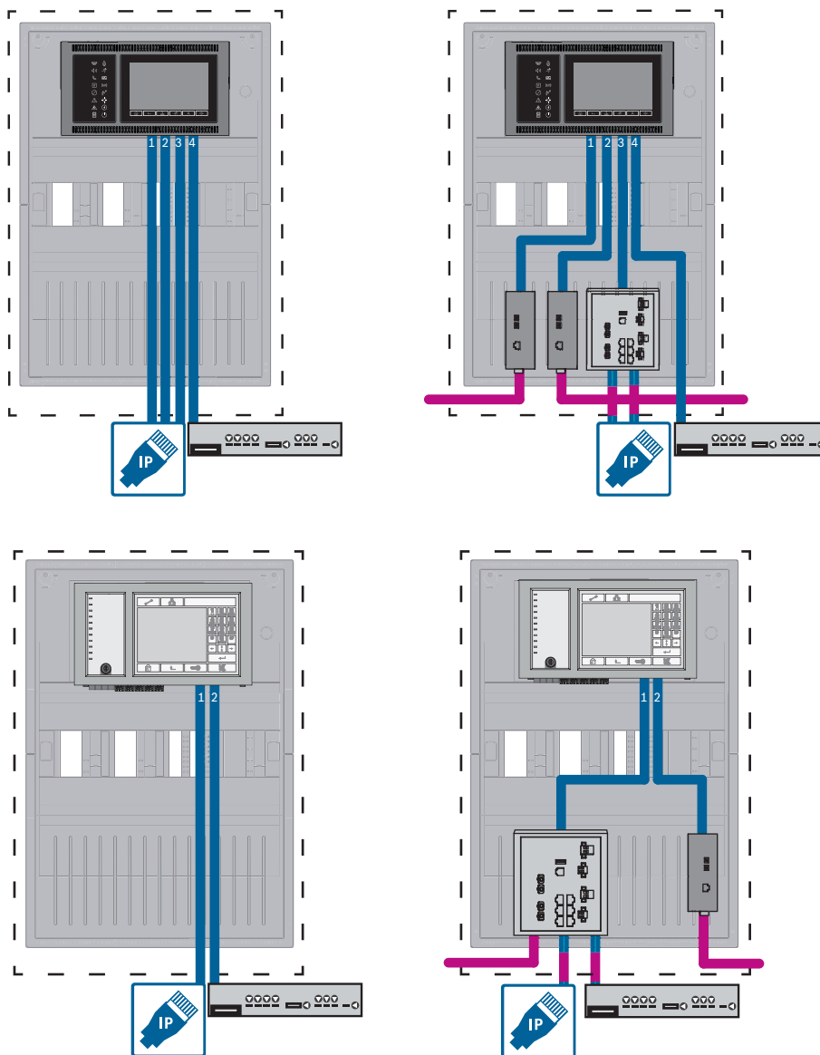
Figura 7.3: Lado izquierdo: sin red de centrales, lado derecho: con la red de centrales Solo se requiere conmutador Ethernet en caso de más de dos servicios conectados a la central.
