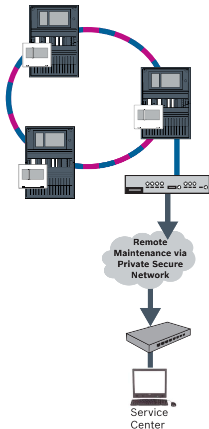
Figura 8.5: Remote Maintenance para una red segura privada
