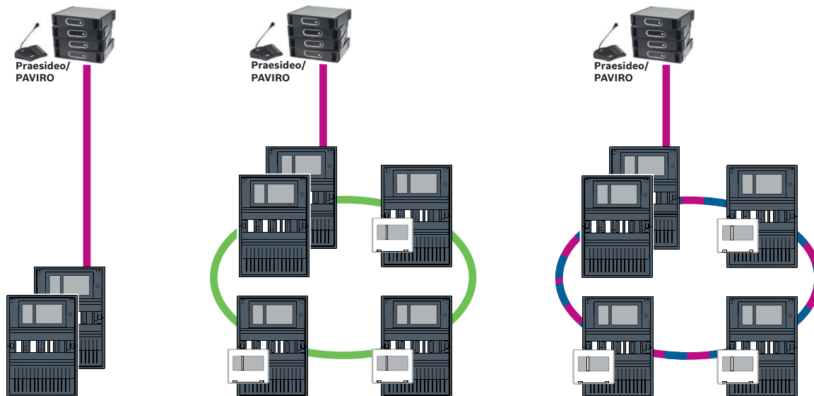
Figura 9.1: Un módulo Praesideo|PAVIRO directo
