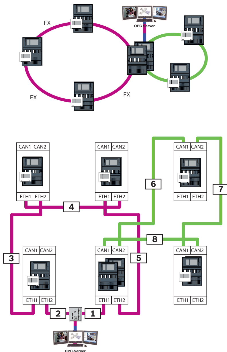
Figura 12.1: Ejemplo de una red y de la numeración de líneas posible
