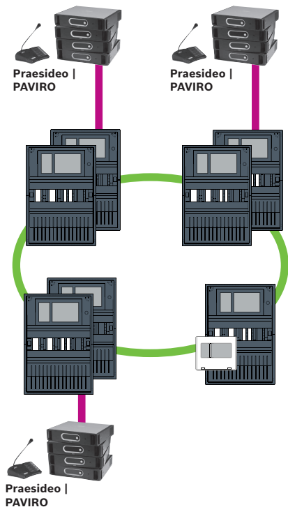
Рис. 9.3: Несколько прямых интерфейсов VAS
