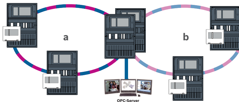
Рис. 4.10: Подключение кольца Ethernet через резервную панель
