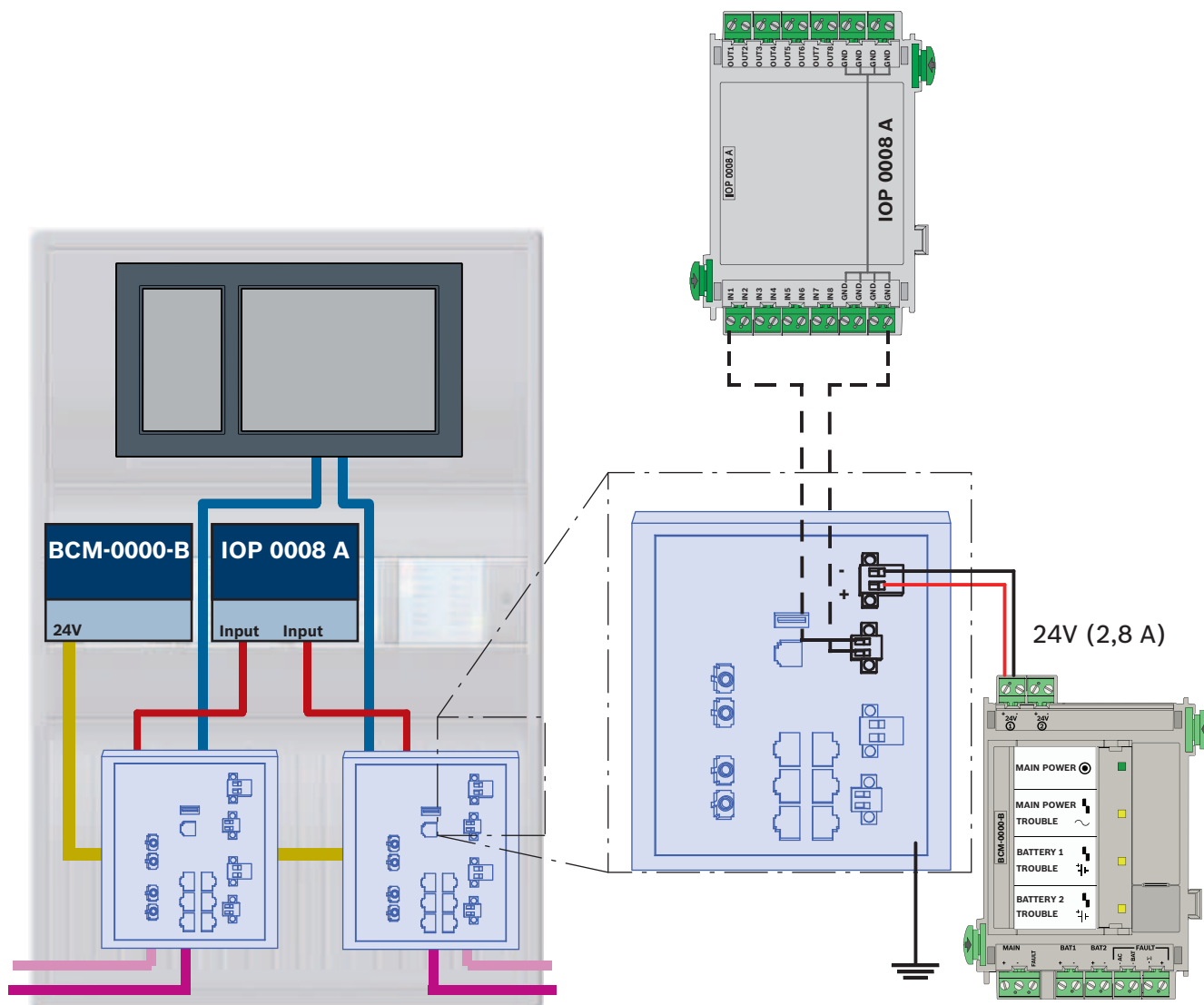
Рис. 11.2: Подключение коммутатора к источнику питания и IOP
