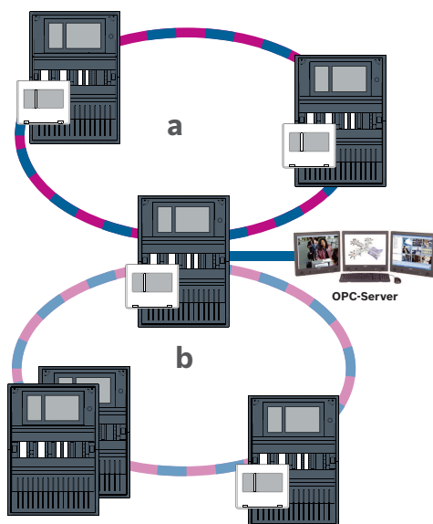
Рис. 4.9: Подключение кольца Ethernet через панель без резервирования
