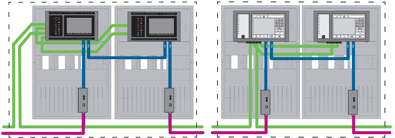
Рис. 7.8: Подключение Ethernet- и CAN-среды с резервными панелями
