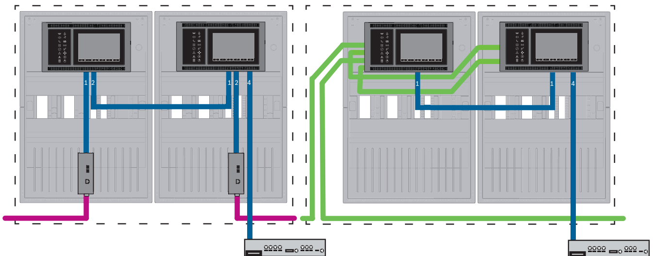
Рис. 7.9: Левая сторона: в сети Ethernet; правая сторона: в сети CAN
