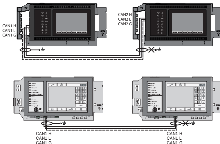
Рис. 6.1: Подключение CAN (вверху: AVENAR, внизу: FPA)
