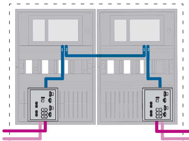
Рис. 7.7: Подключение Ethernet-сетей с резервными панелями
