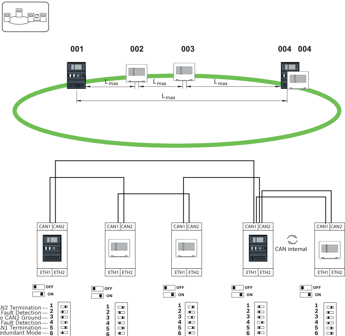
Рис. 10.5: Настройки DIP-переключателя для кольцевой топологии с удаленной клавиатурой (только AVENAR)
