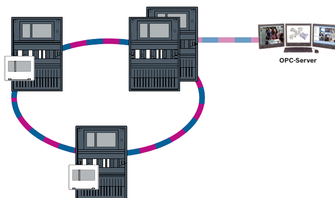
Рис. 4.5: Кольцо Ethernet с OPC-сервером к резервной панели
