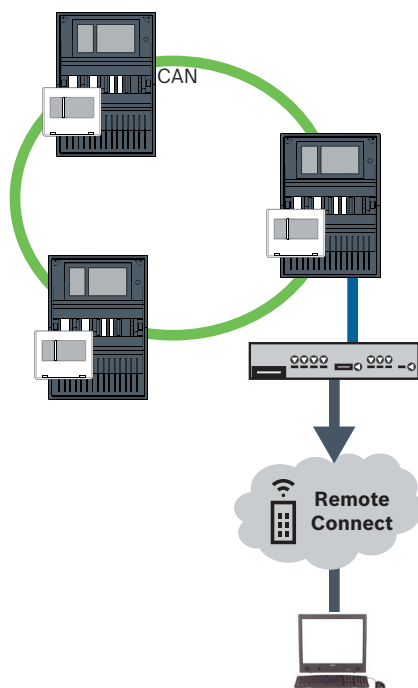
Рис. 8.2: Remote Connect в кольце CAN
