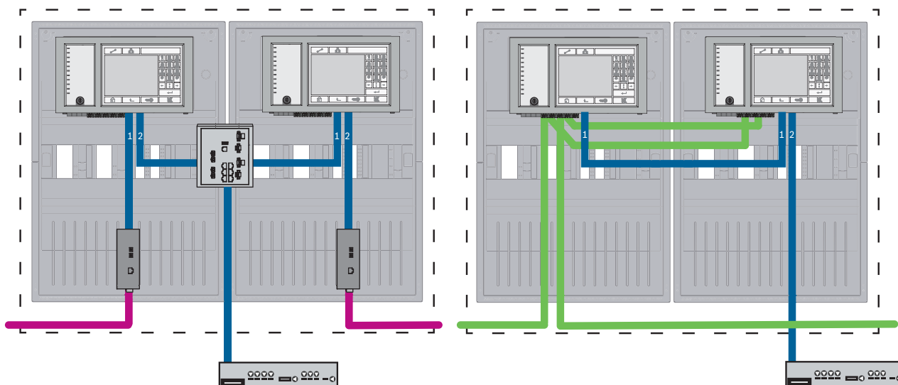
Рис. 7.10: Левая сторона: в сети Ethernet; правая сторона: в сети CAN
