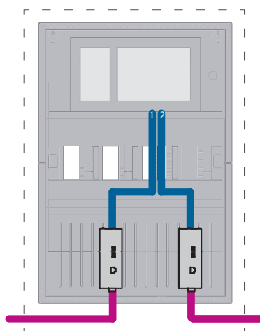
Рис. 7.1: Ethernet-сеть панелей
