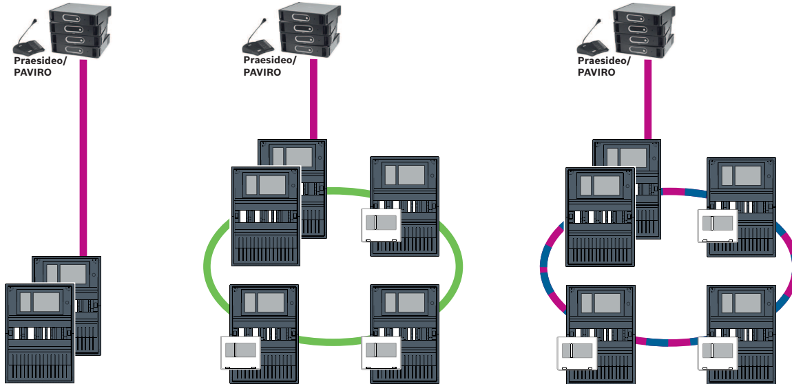
Рис. 9.1: Один прямой интерфейс Praesideo|PAVIRO
