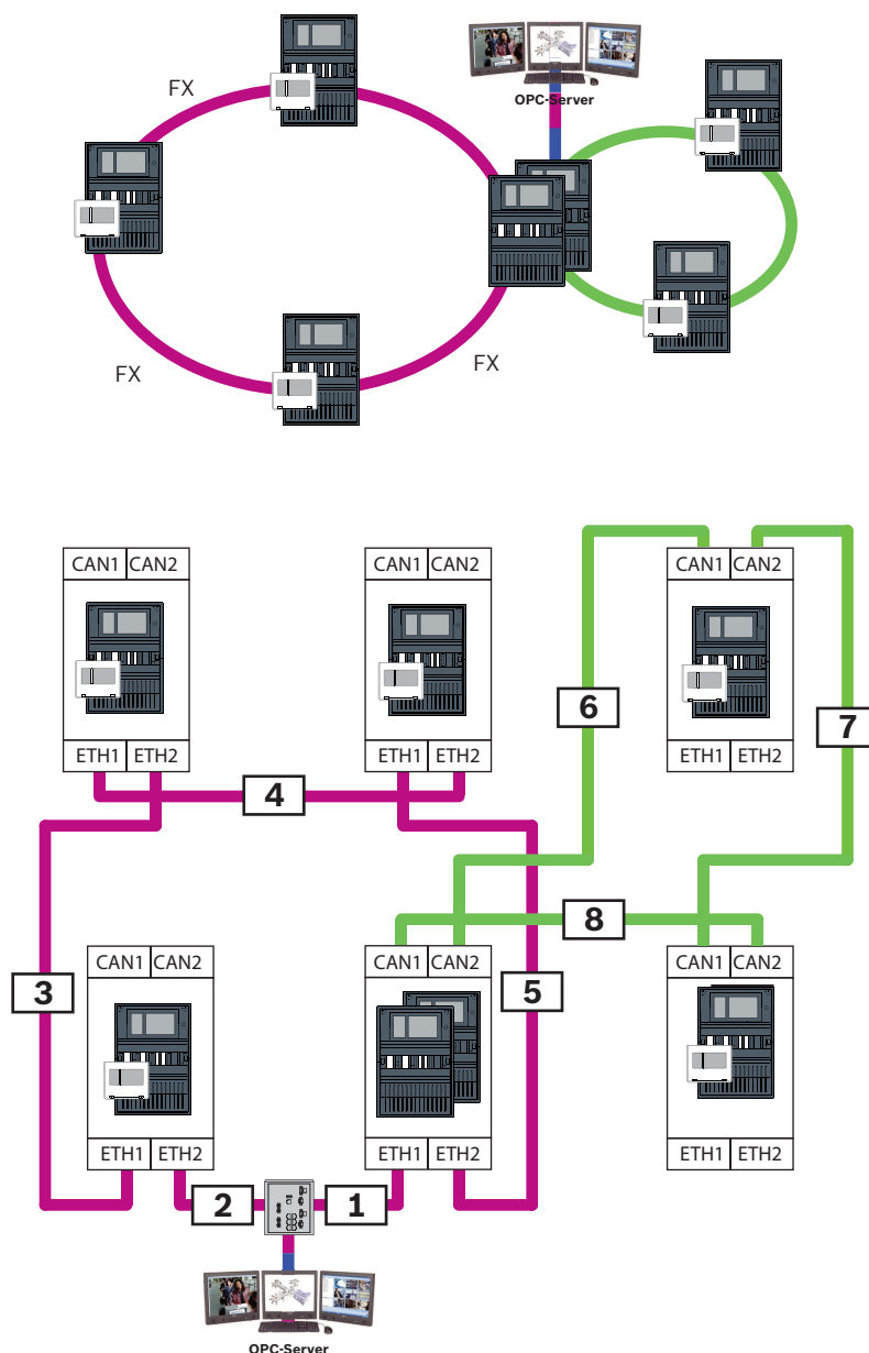
Рис. 12.1: Пример сети и возможной нумерации линий
