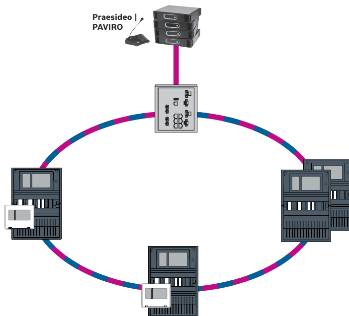
Рис. 9.4: VAS, интегрированная в Ethernet сеть панелей
