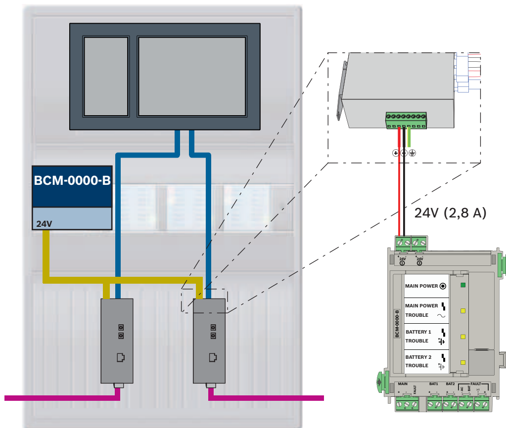
Рис. 11.1: Подключение преобразователя среды к источнику питания и к входу IN1/IN2 контроллера панели
