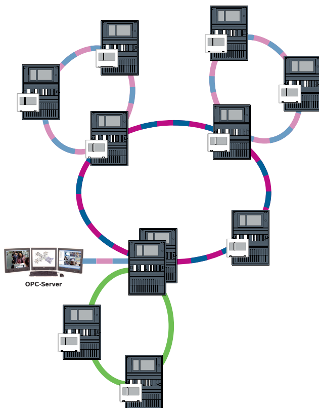
Рис. 4.8: Магистраль Ethernet с кольцевыми подсетями
