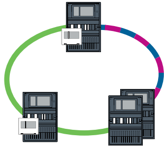
Рис. 4.7: Кольцо CAN с сегментами Ethernet
