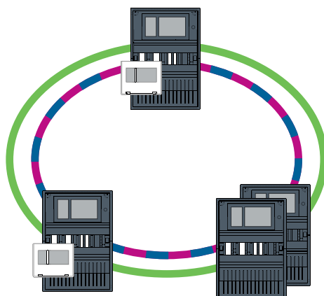
Рис. 4.6: Двойное кольцо Ethernet и CAN
