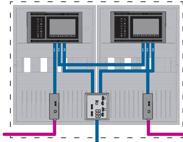
Рис. 7.11: Интерфейс для подключения VAS и иерархической панели к резервной панели AVENAR
