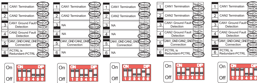
Рис. 10.4: Настройки DIP-переключателей для кольцевой топологии с резервными панелями (вверху: AVENAR, внизу: FPA)
