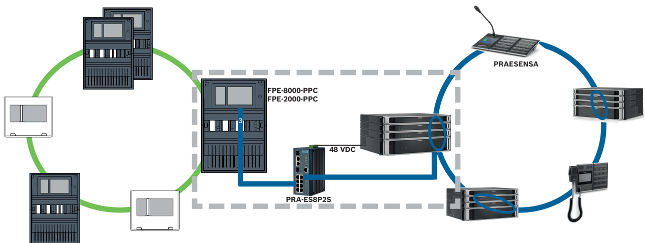
Рис. 9.2: Подключение PRAESENSA к панели AVENAR
