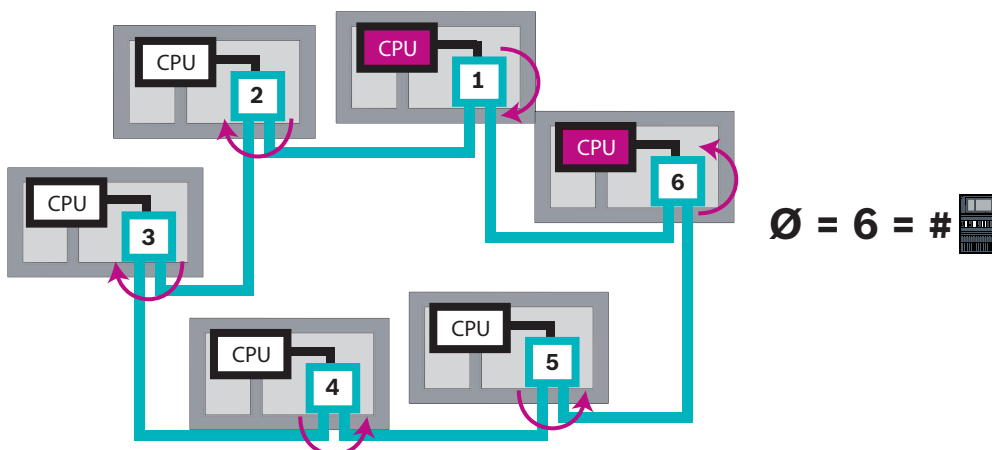
Рис. 5.2: Сетевой диаметр кольца с 6 панелями
