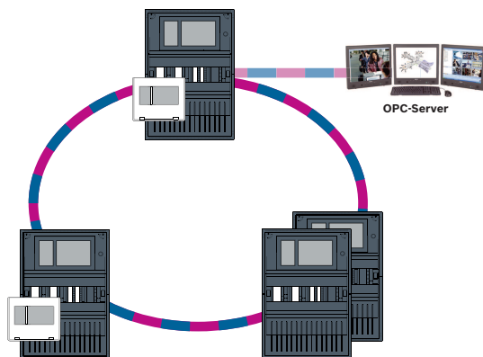
Рис. 4.4: Кольцо Ethernet с OPC-сервером
