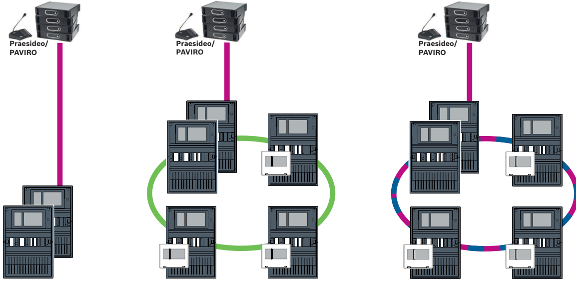
Şekil 9.1: Tek doğrudan Praesideo|PAVIRO arayüzü
