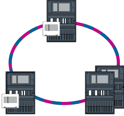
Şekil 4.3: Ethernet döngüsü
