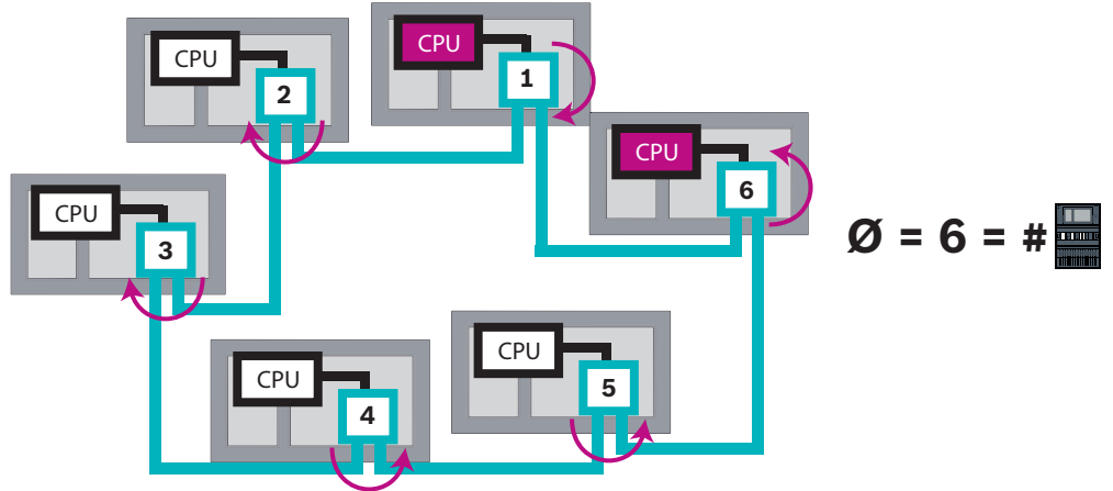
Şekil 5.2: 6 panel bulunan bir döngünün ağ çapı
