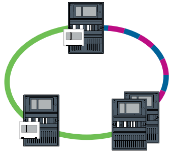
Şekil 4.7: Ethernet segmentlerine sahip CAN döngüsü
