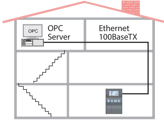
Şekil 4.1: OPC sunucusu aracılığıyla BIS'ye bağlantı
