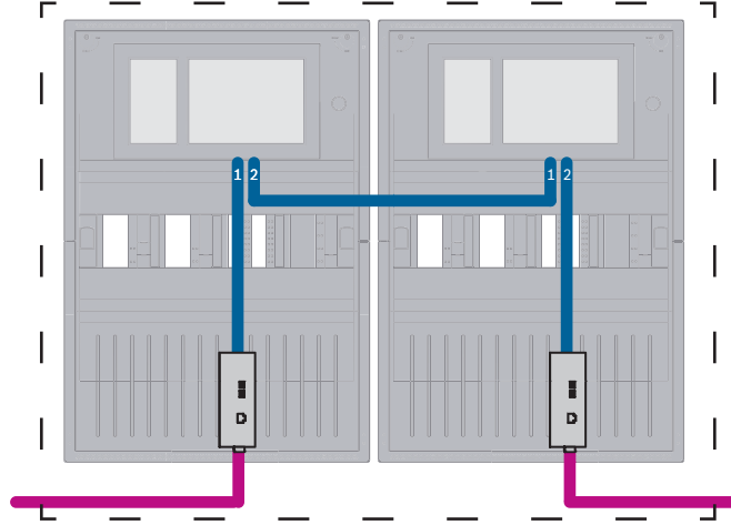
Şekil 7.4: Yedek panellerle Ethernet üzerinden panel ağı 100 m'den büyük aralıklar için medya dönüştürücüler ile aralığı uzatmak zorunludur. 100 m'den küçük aralıklar için medya dönüştürücüler gerekli olmayabilir.
