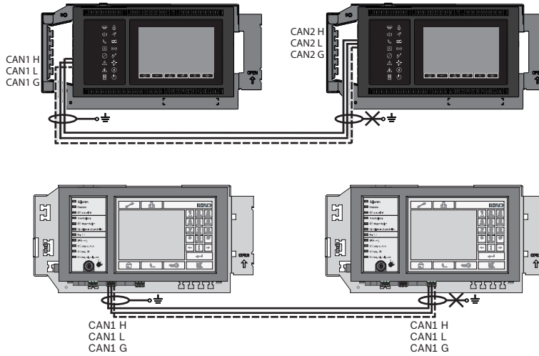
Şekil 6.1: CAN bağlantısı (üst: AVENAR, alt: FPA)
