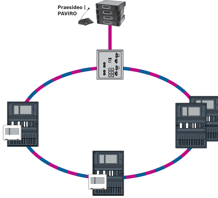
Şekil 9.4: Ethernet panel ağına entegre VAS
