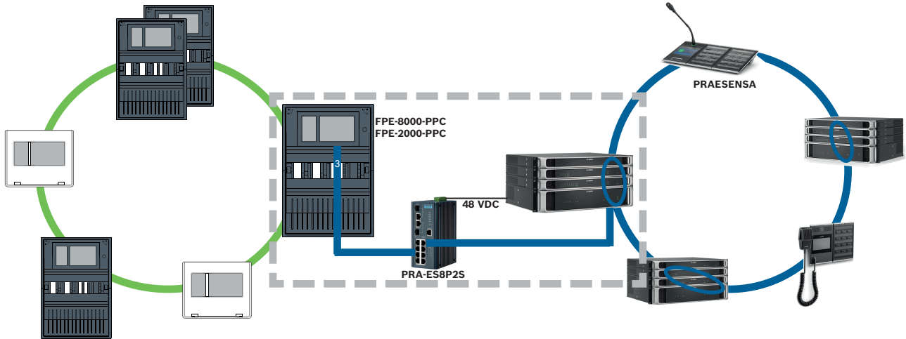
Şekil 9.2: PRAESENSA'dan AVENAR panele
