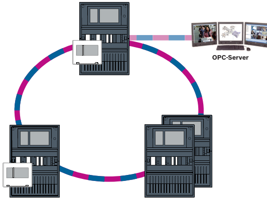
Şekil 4.4: OPC sunuculu Ethernet döngüsü
