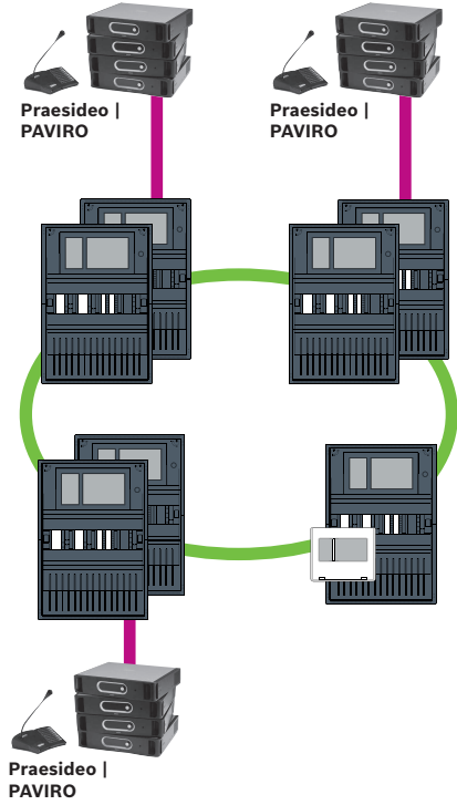
Şekil 9.3: Birden çok doğrudan VAS arayüzü
