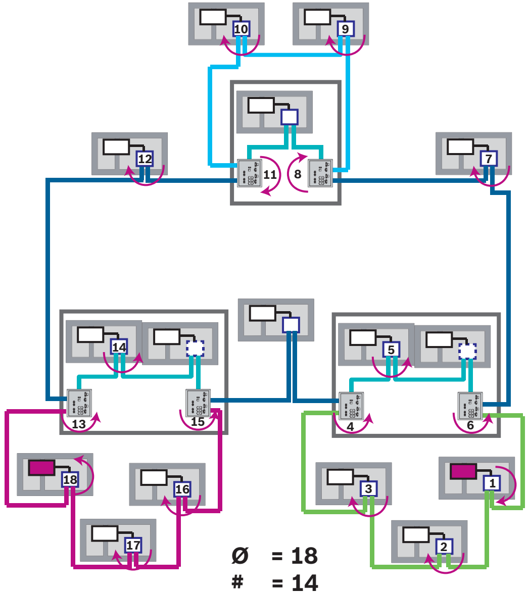
Şekil 5.3: Alt döngüler bulunan ana iletişim hattının ağ çapı
