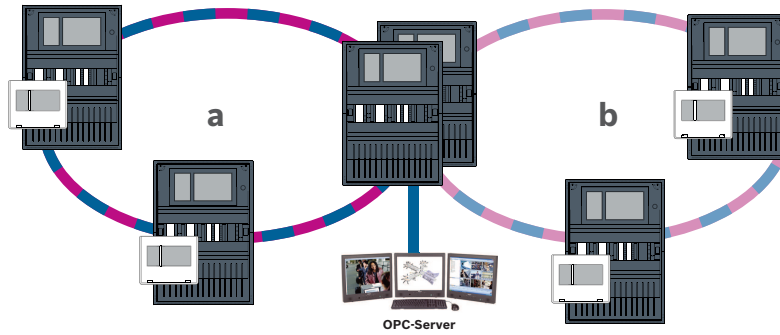
Şekil 4.10: Yedek panel aracılığıyla Ethernet döngüsünü bağlama
