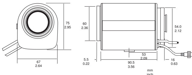
Abmessungen LTC 3283/40
