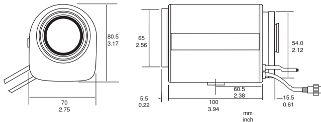
Abmessungen LTC 3283/50
