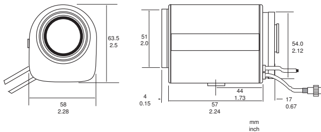
Abmessungen LTC 3283/20
