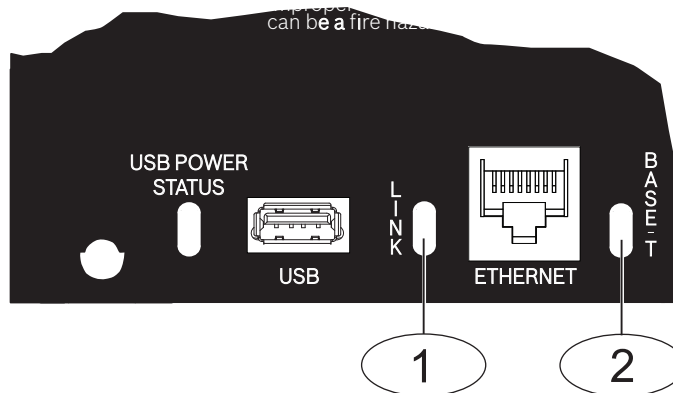
Afbeelding 8.1: Ingebouwd ethernet en leds
