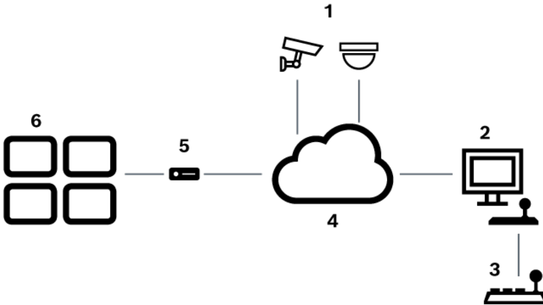
Attēls 5.1: 1. scenārijs: Bosch IntuiKey tastatūra, kas savienota ar Bosch Video Management System darbstaciju
