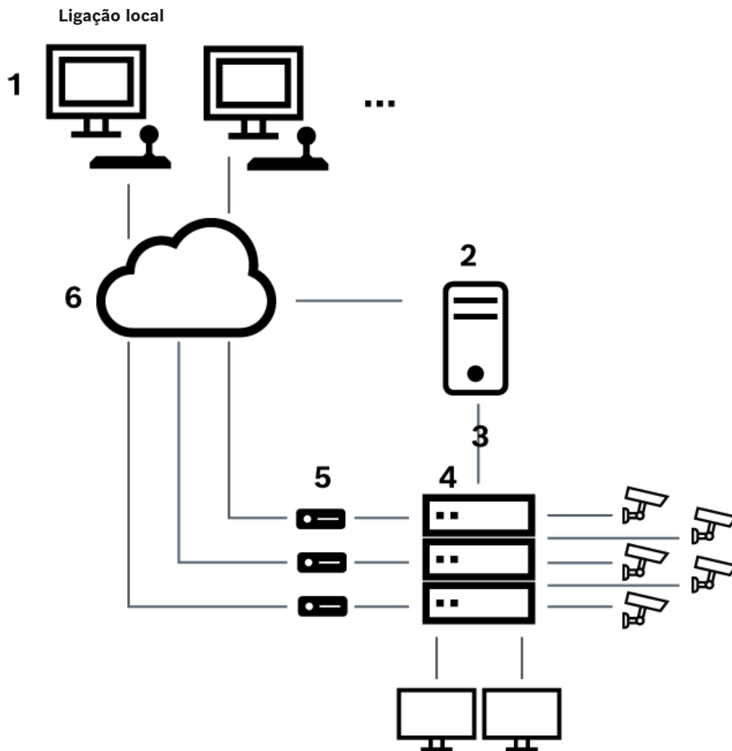
Figura 5.3: Ligação local do Bosch Video Management System a um comutador matricial Allegiant Bosch
