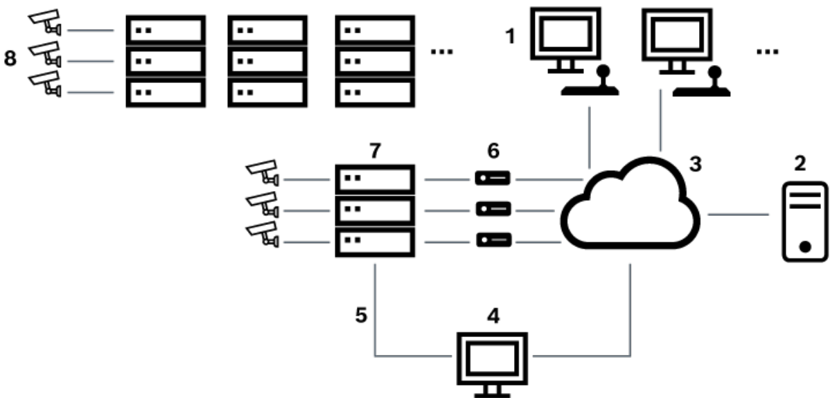
Figura 5.5: Sistema Allegiant Bosch ampliado com computadores Satélite
