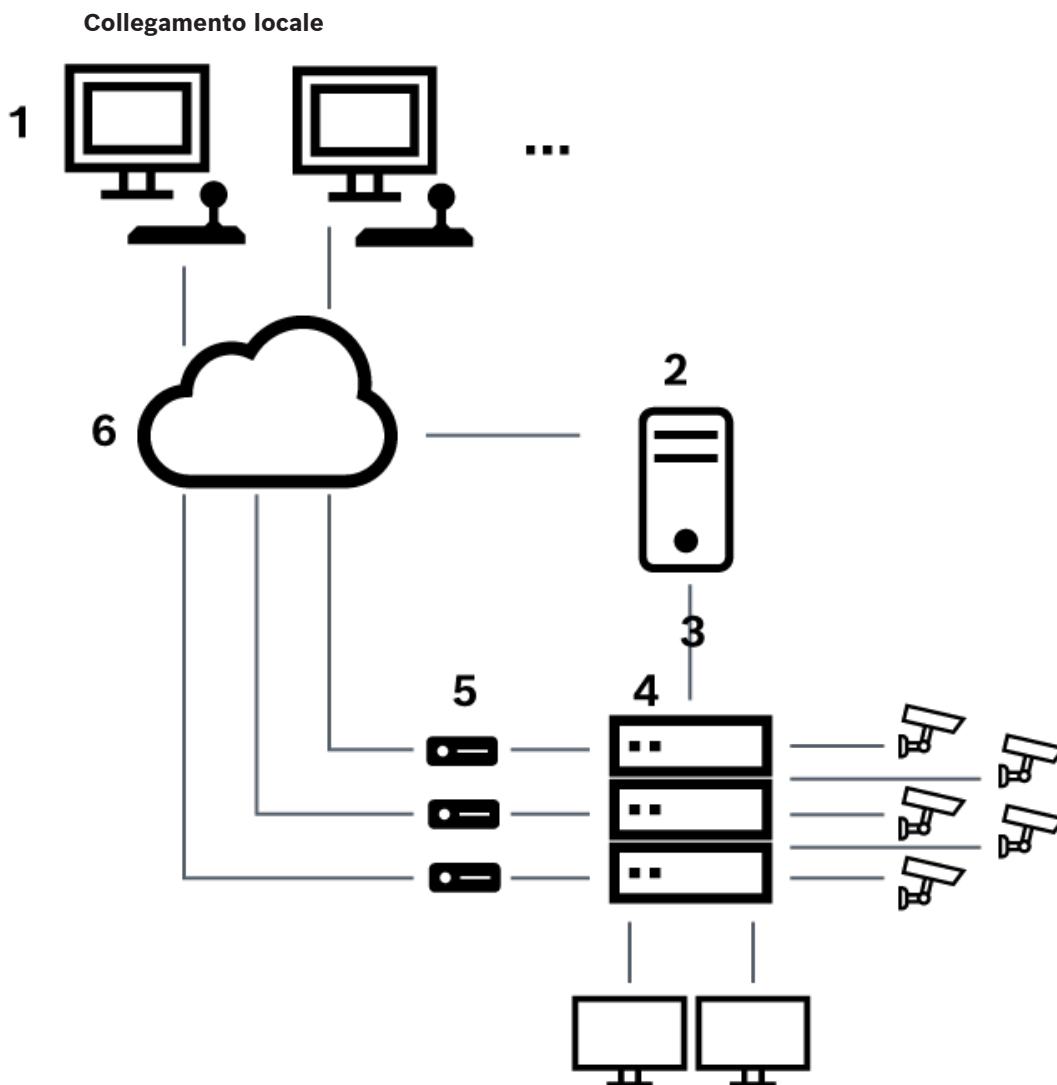
Figura 5.3: Collegamento locale di Bosch Video Management System ad una matrice Bosch Allegiant
