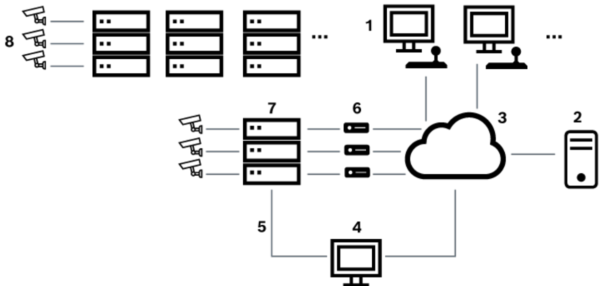
Afbeelding 5.5: Bosch Allegiant-systeem uitgebreid met satellietschakelaars
