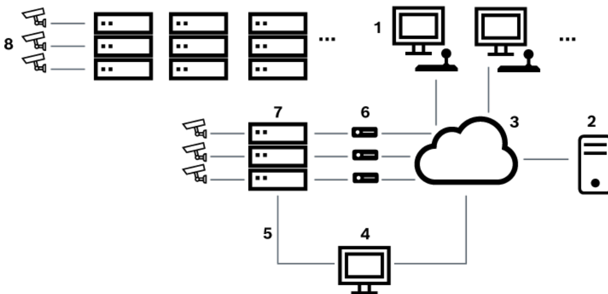
Рис. 5.5: Система Bosch Allegiant, расширенная за счет спутниковых коммутаторов
