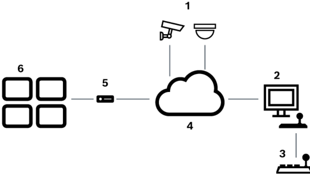
그림 5.1: 시나리오 1: Bosch Video Management System 워크스테이션에 연결된 Bosch IntuiKey 키보드
