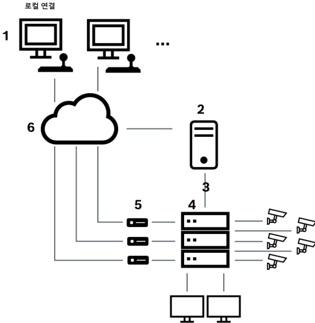
그림 5.3: Bosch Allegiant 매트릭스 스위치에 대한 Bosch Video Management System 로컬 연결
