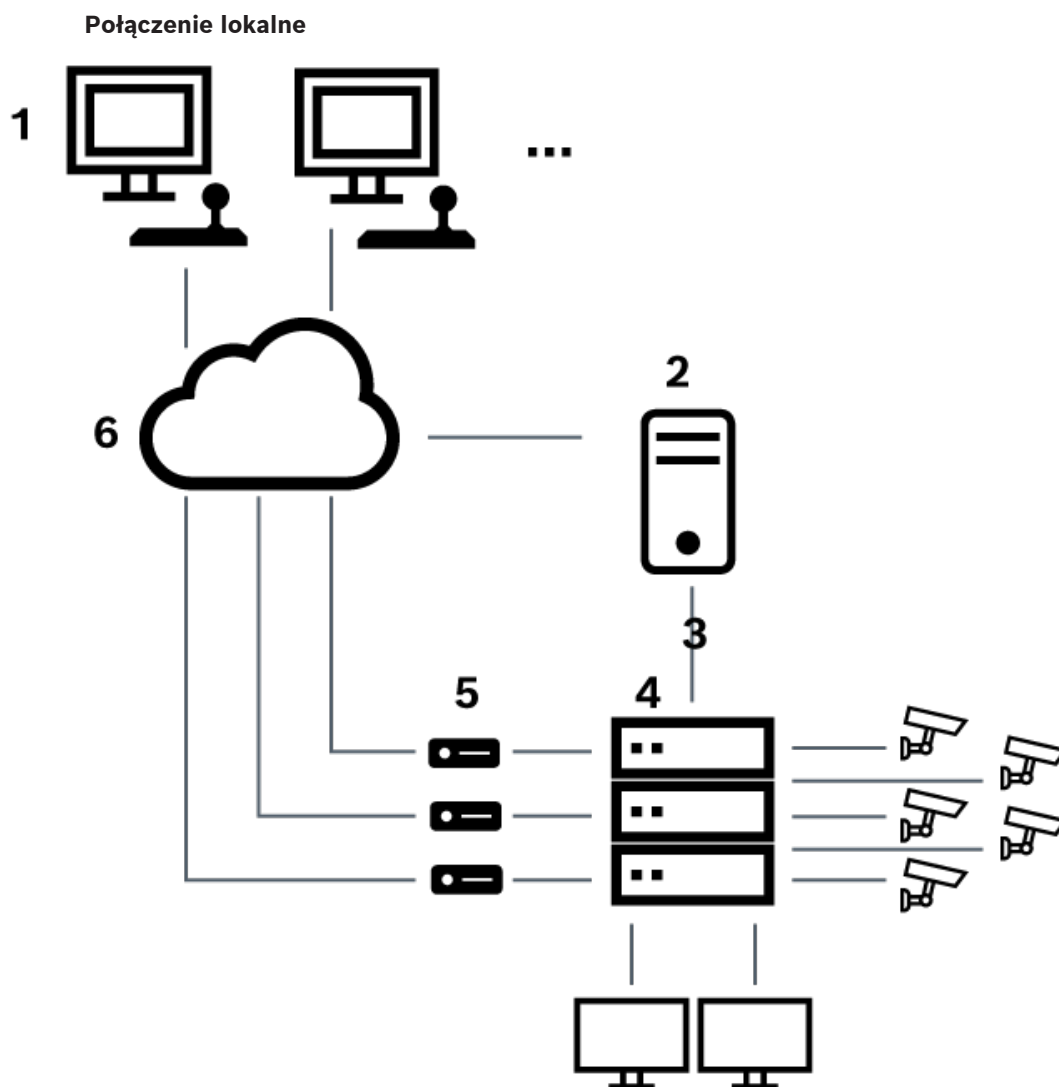
Rysunek 5.3: Lokalne połączenie systemu BVMS z krosownicą Bosch Allegiant
