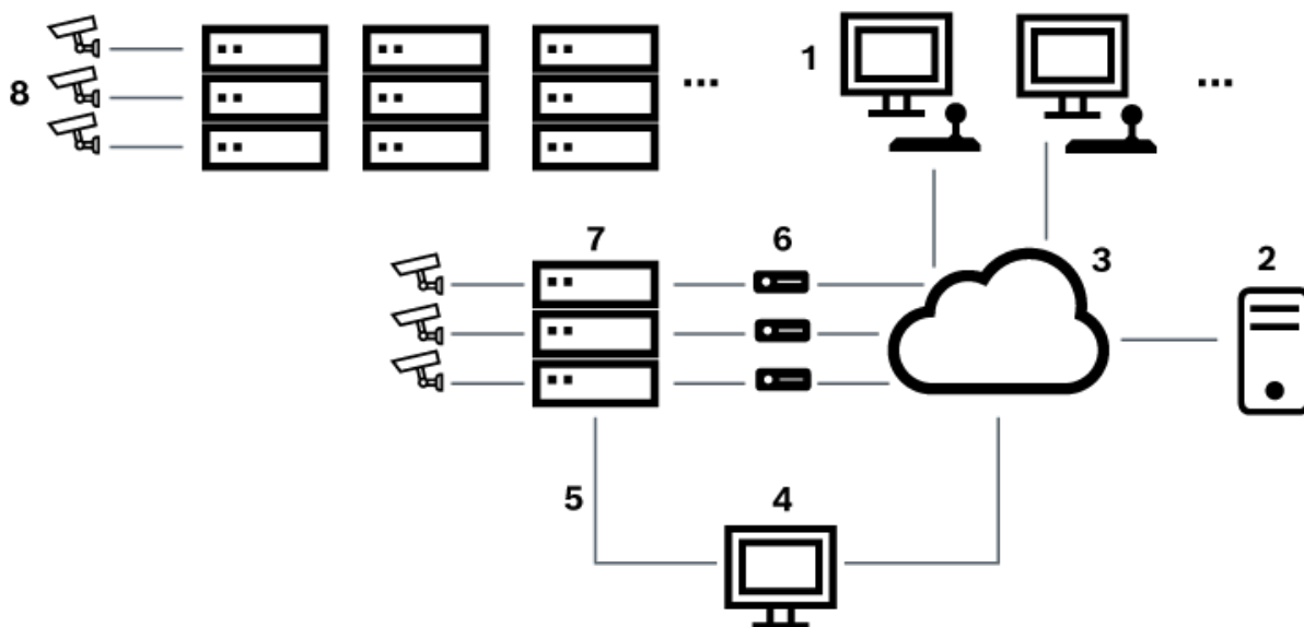
图片 5.5: 使用子网切换扩展 Bosch Allegiant 系统
