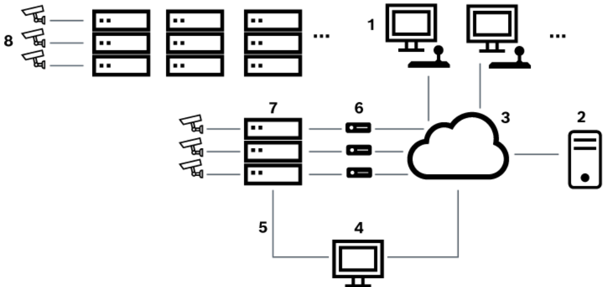
Vyobrazení 6.5: Systém Bosch Allegiant rozšířený satelitními přepínači
