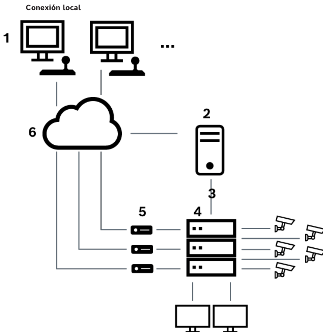
Figura 6.3: Conexión local de Bosch Video Management System a una matriz Allegiant de Bosch
