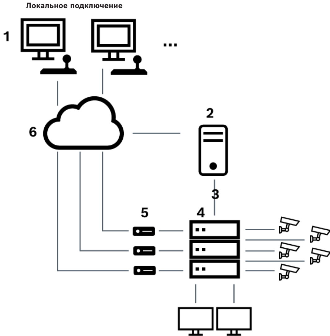
Рис. 6.3: Локальное подключение Bosch Video Management System к матричному коммутатору Bosch Allegiant
