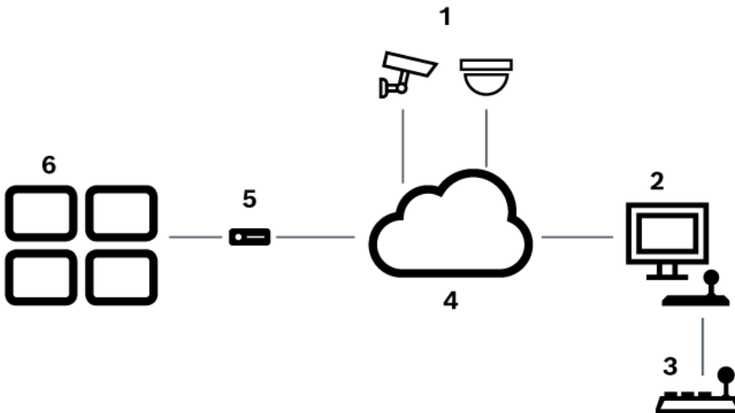
Рис. 6.1: Сценарий 1: клавиатура Bosch IntuiKey, подключенная к рабочей станции Bosch Video Management System
