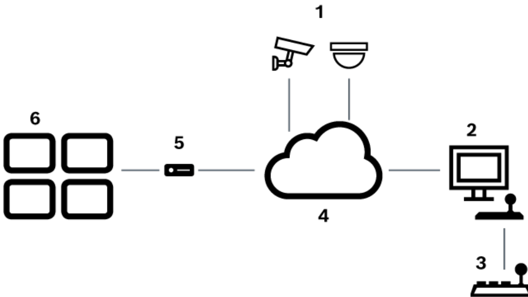
Figur 6.1: Scenario 1: Bosch IntuiKey-tangentbord anslutet till en Bosch Video Management System-arbetsstation
