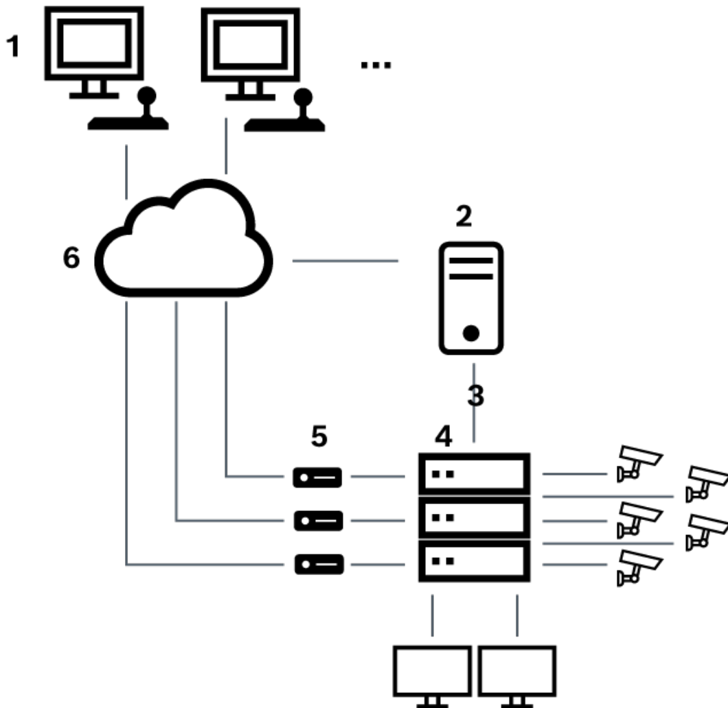
Abbildung 6.3: Lokale Verbindung des Bosch Video Management System mit einem Bosch Allegiant-Matrix-Switch
