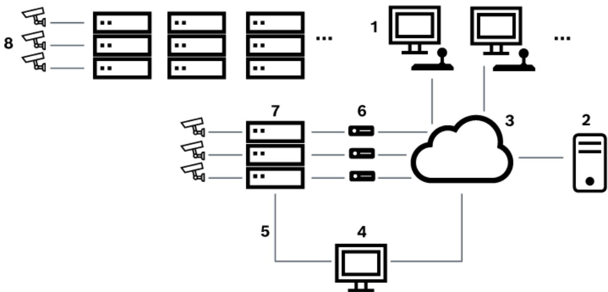
Abbildung 6.5: Mit Satellitenkreuzschienen erweitertes Bosch Allegiant System
