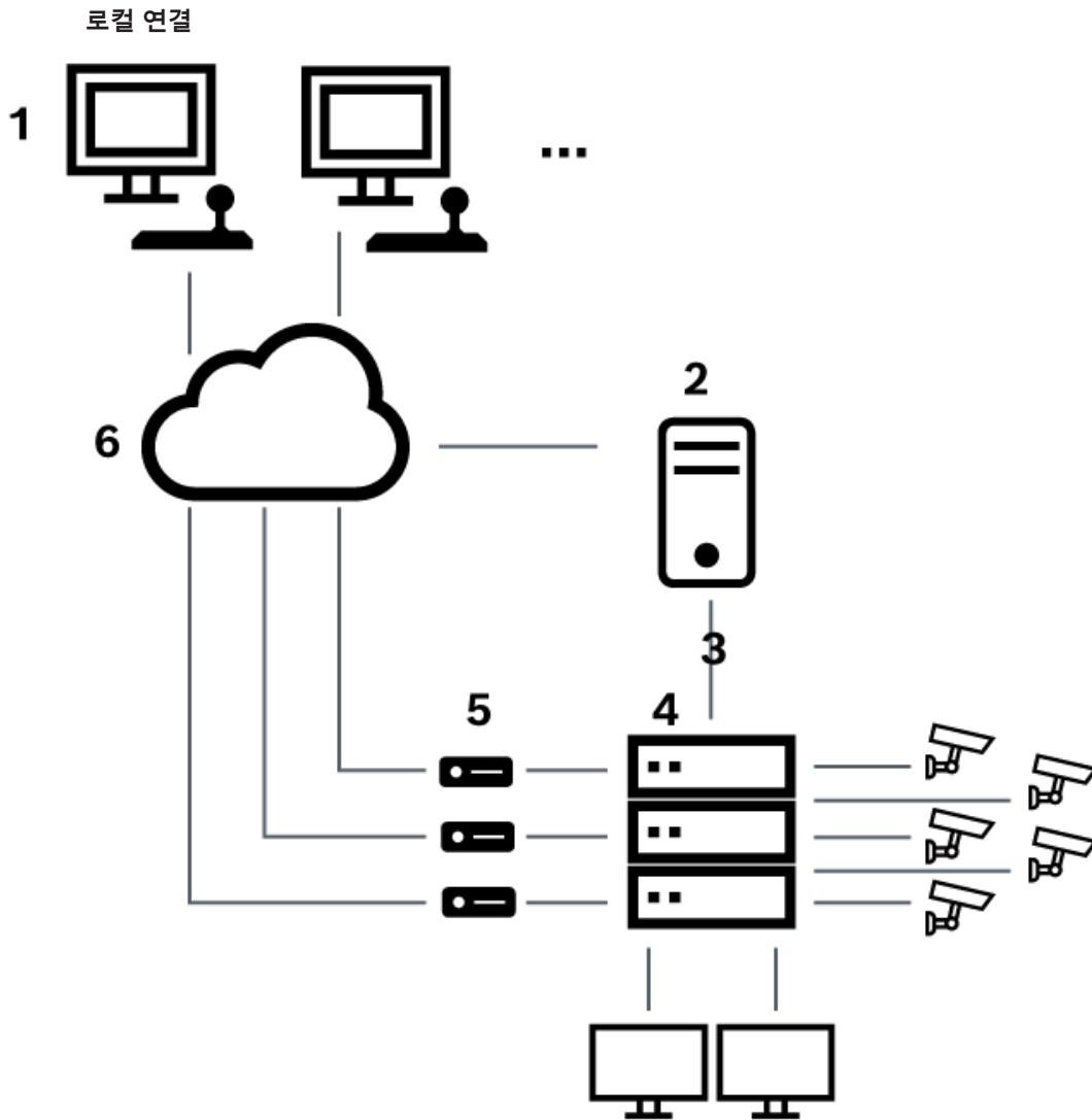
그림 6.3: Bosch Allegiant 매트릭스 스위치에 대한 Bosch Video Management System 로컬 연결
