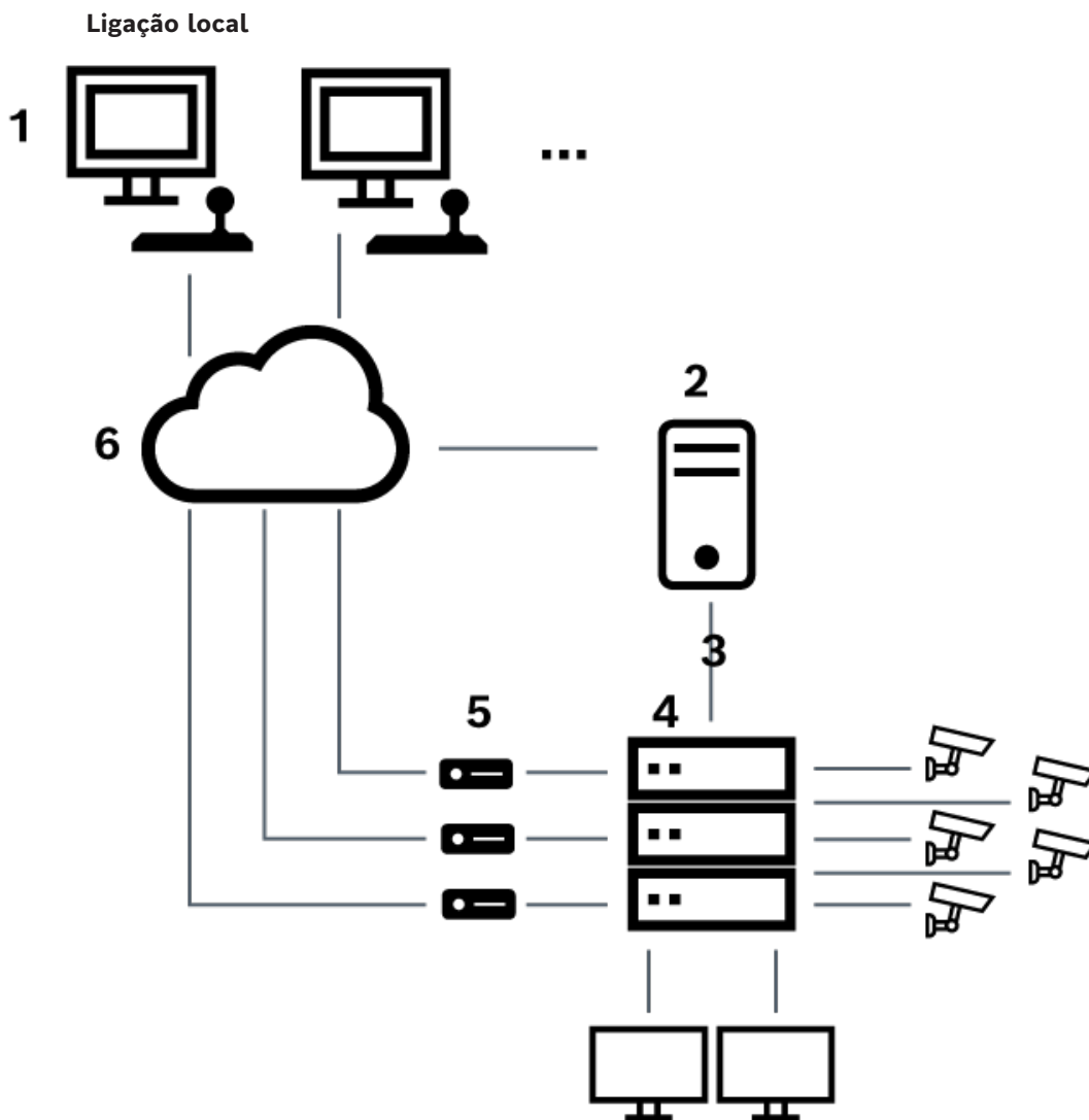
Figura 6.3: Ligação local do Bosch Video Management System a um comutador matricial Allegiant Bosch
