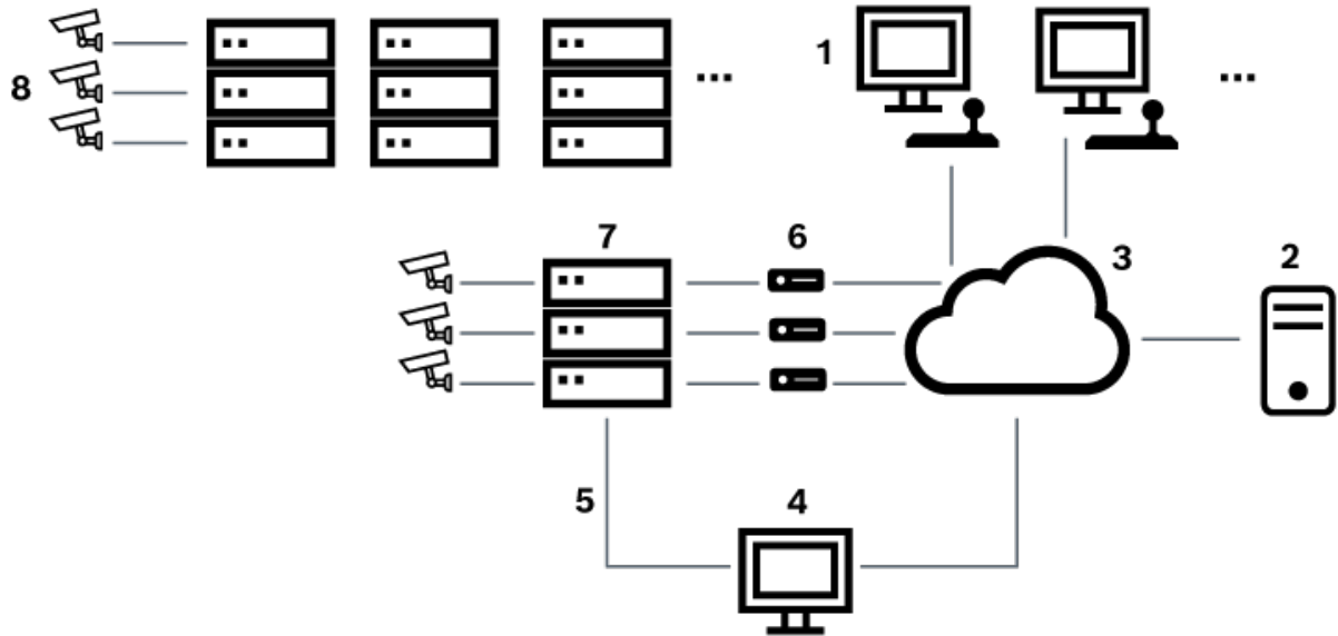
图片 6.5: 使用子网切换扩展 Bosch Allegiant 系统
