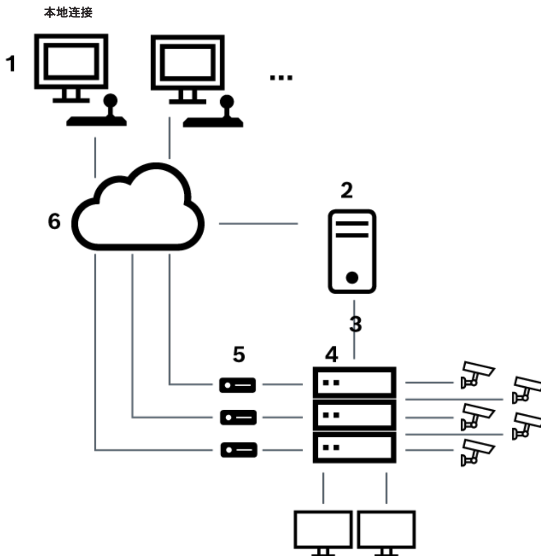
图片 6.3: Bosch Video Management System 与 Bosch Allegiant 矩阵切换台的本地连接
