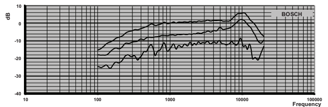
Afb. 1: Frequentiebereik (openingshoek: 0, 90 en 180 graden)
