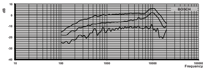
圖 1: 頻率響應 (開啟角度: 0、90 和 180 度)
