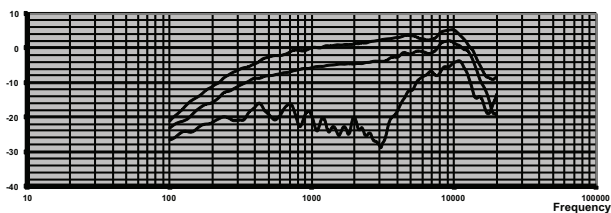
Kuva 1: Taajuusvaste (avauskulma: 0, 90 ja 180 astetta)
