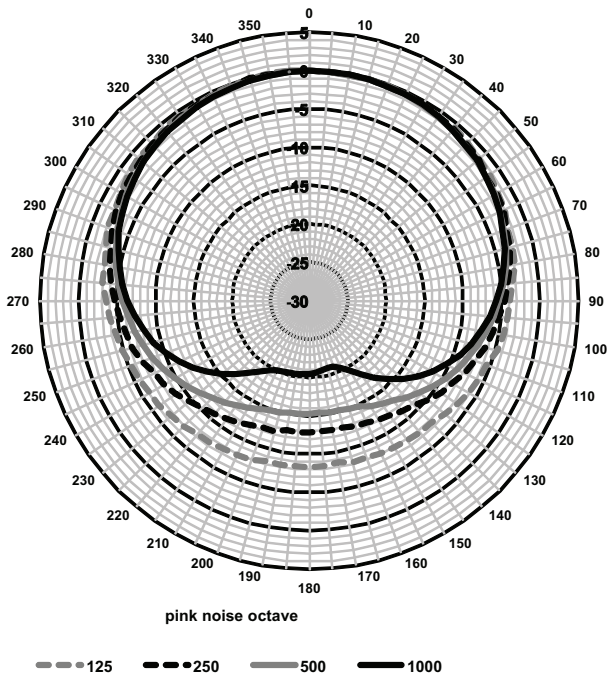
Gbr. 2: Diagram kutub (diukur dengan pink noise)
