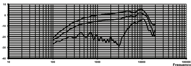
Gbr. 1: Respons frekuensi (Sudut bukaan: 0, 90 dan 180 derajat)
