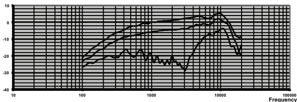
Hình 1: Đáp ứng tần số (Góc mở: 0, 90 và 180 độ)
