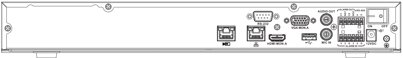
Fig. 1: Panel posterior del DIVAR network 2000 (sin PoE)
