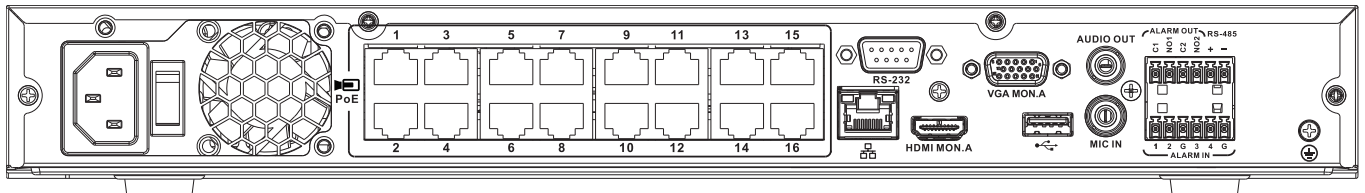
Fig. 3: Panel posterior del DIVAR network 2000 (16 PoE)
