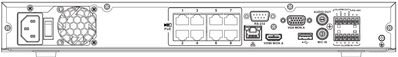
Fig. 2: Panel posterior del DIVAR network 2000 (8 PoE)
