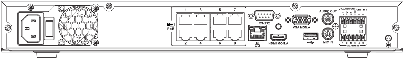
图片 2: DIVAR2000网络 (8 PoE) 后面板
