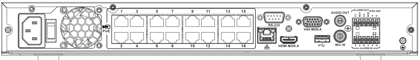
图片 3: DIVAR2000网络(16 PoE)后面板
