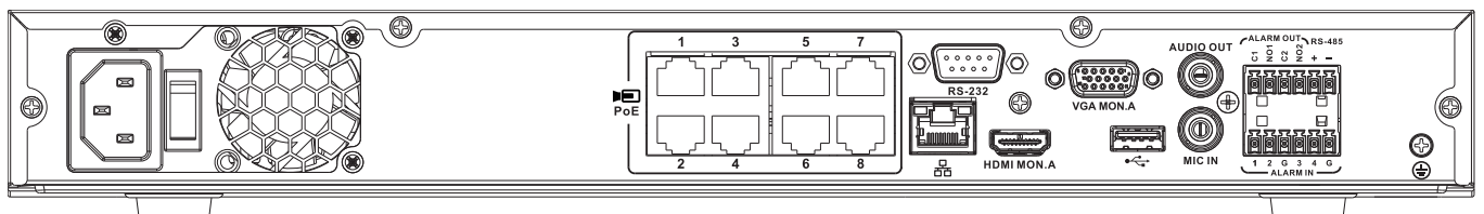
圖 2: DIVAR network 2000 (8 PoE) 後方面板
