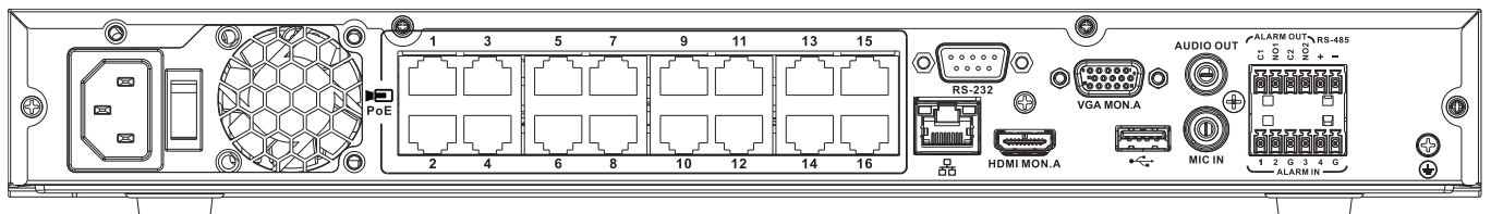
圖 3: DIVAR network 2000 (16 PoE) 後方面板
