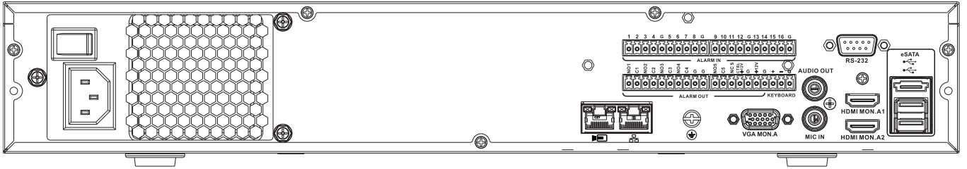
图片 1: DIVAR 5000网络后面板 (无PoE)
