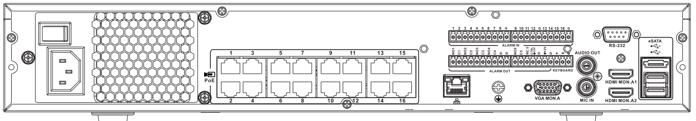
DIVAR 5000网络后面板(16 PoE)
