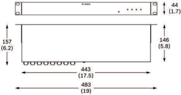
Abb. 1: Abmessungen (in mm/Zoll)
