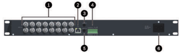
Εικ. 3: Πίσω όψη VIDEOJET multi 4000
