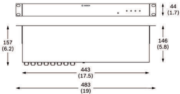
Fig. 1: Dimensiones en mm (pulg.)
