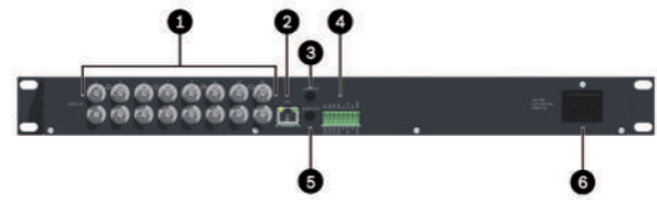
Fig. 3: Parte posterior de VIDEOJET multi 4000
