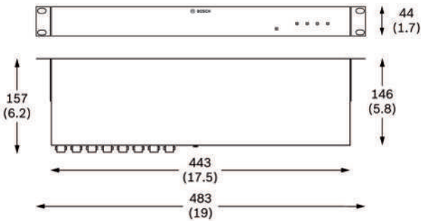
Ábra 1: Méretetek mm-ben
