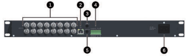
Ábra 3: VIDEOJET multi 4000 hátulnézet
