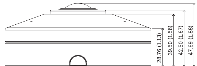
Dimensiones en mm (pulgadas)
