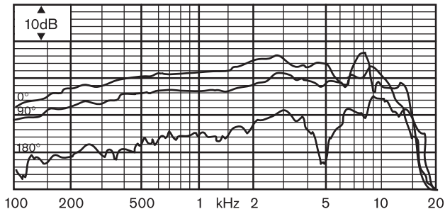
Απόκριση συχνότητας
