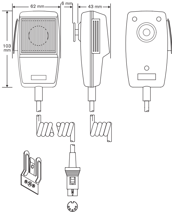
Mitat millimetreinä
