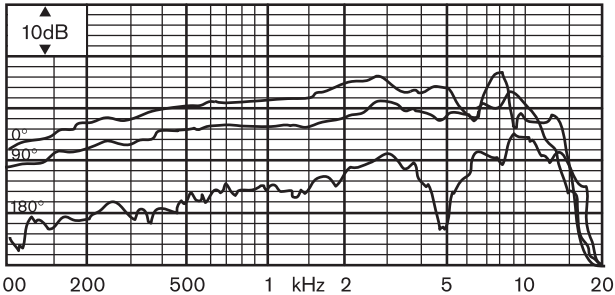
Taajuusvaste
