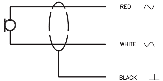
Devre şeması
