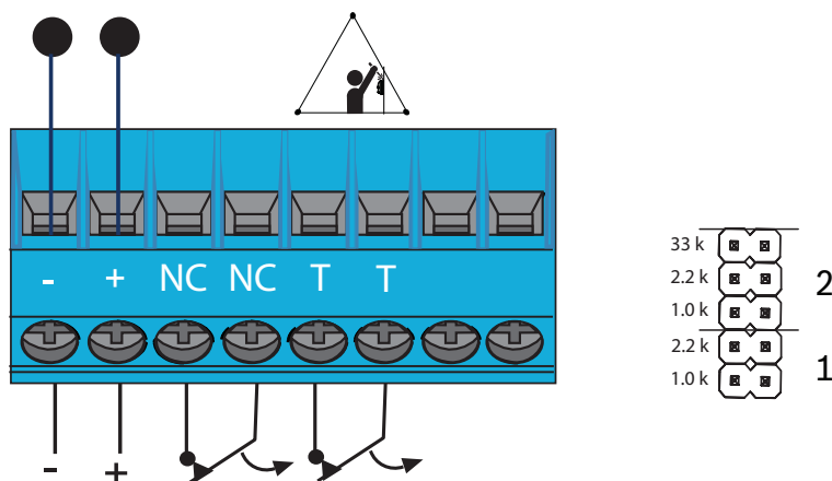
Figur 6.2: Ändmotstånd – översikt
