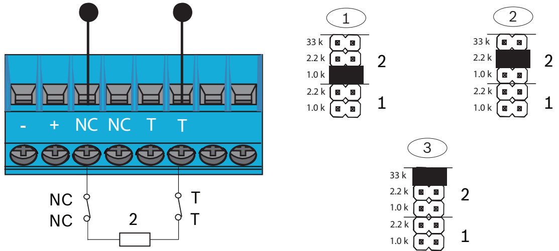
Figur 6.5: Enkelbalanserad slinga
