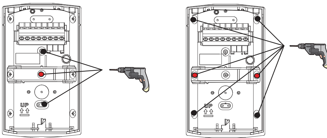
Figur 5.3: Vänster: vägmontering, höger: hörnmontering
