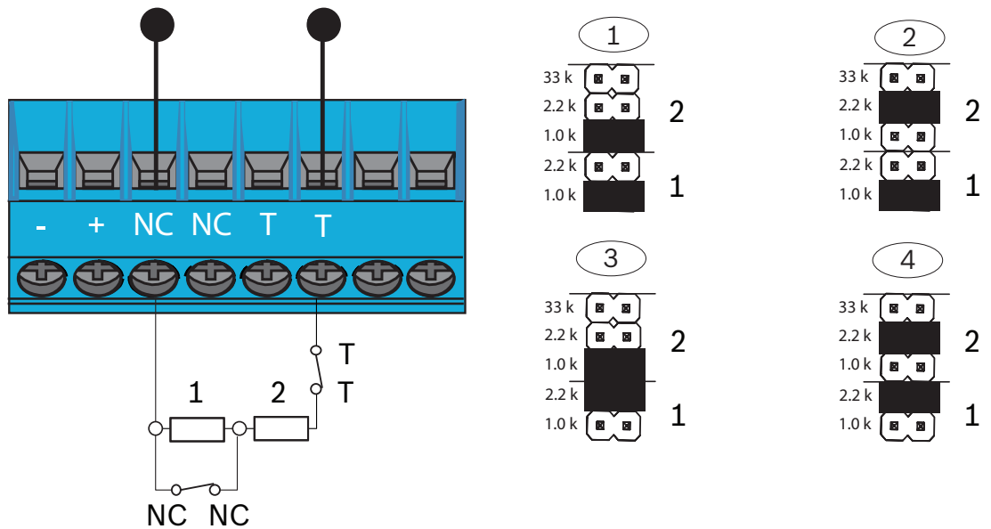
Figur 6.6: Dubbelbalanserad slinga
