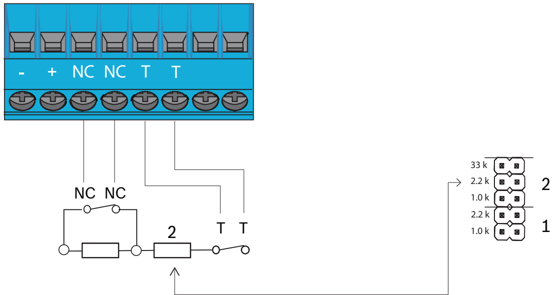
Figur 6.4: Sabotageskyddsmotstånd - översikt
