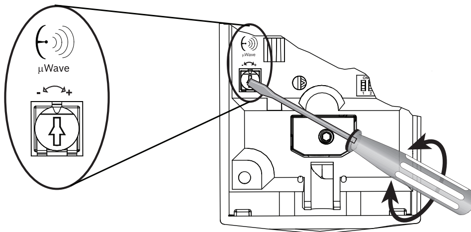
Figur 7.4: Potentiometer för justering av mikrovågor
