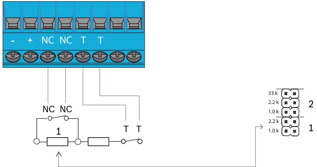
Figur 6.3: Larmmotstånd – översikt
